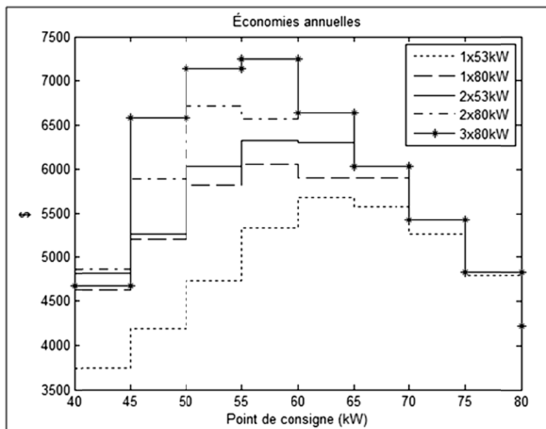
Figure 2.6 Économies annuelles Centech, première itération
