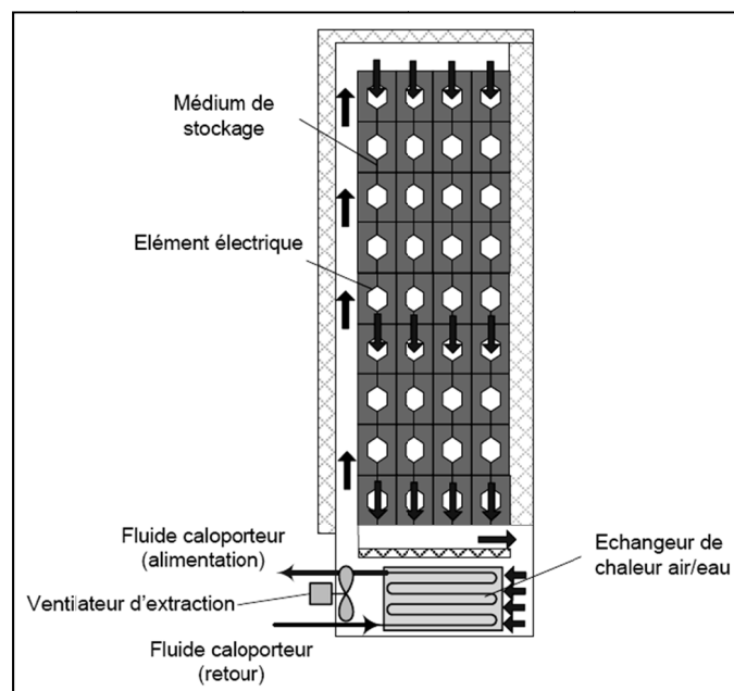
Figure 1.6 Schéma du ThermElect ® hydronique (Moreau, 2010)
