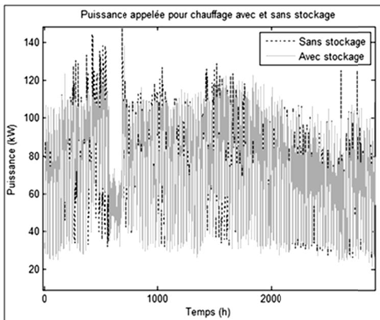
Figure 2.10 Puissance appelée totale du Centech avec et sans stockage
