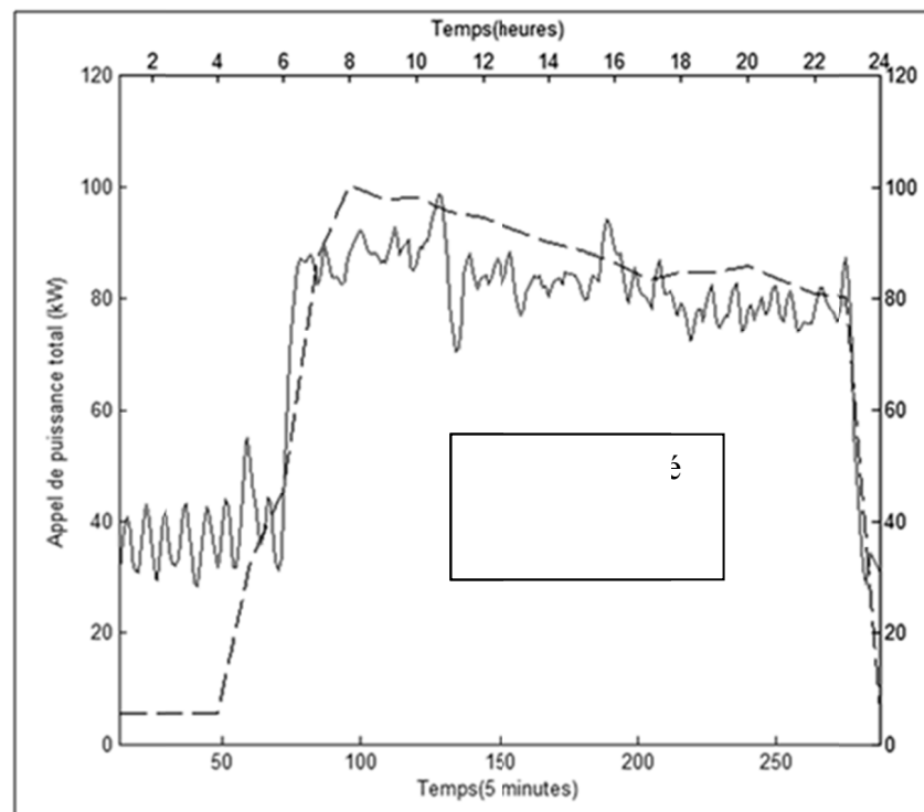
Figure 2.15 Comparaison de profil d'appel de puissance totale entre Simeb ® et les données enregistrées du Centech
