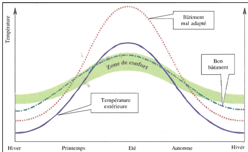
Figure 2.4 Évolution des températures dans des bâtiments au cours de l'année, en absence de chauffage ou de climatisation
