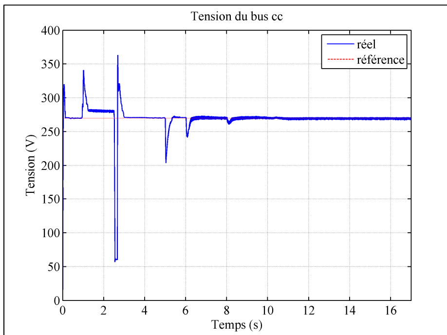
Figure 4.11 Tension réelle et référence au bus cc lors de la simulation dans un aéronef de type Bombardier CRJ
