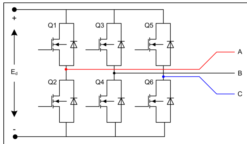
Figure 3.28 Schéma explicatif de l'onduleur
