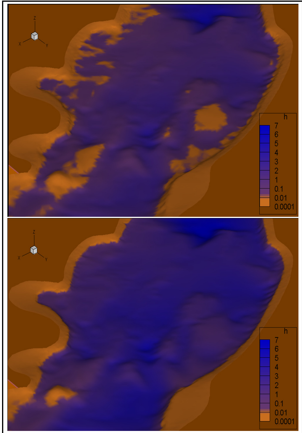
Figure 3.25 Rivière des Prairies Vue 3-D des bancs couvrants-découvants après 1200 s et 2700 s
