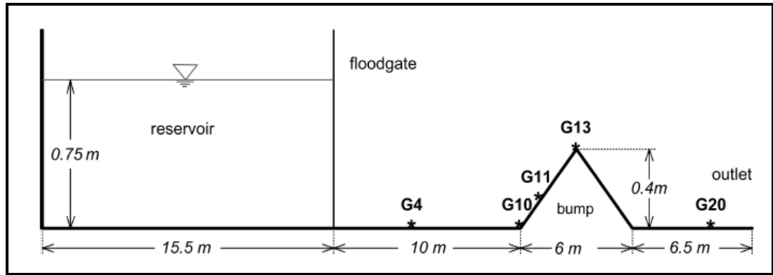
Figure 3.8 CADAM Test 2. Réservoir et canal avec obstacle triangulaire Tirée de Loukili et Soulimani (2007, p. 82)
