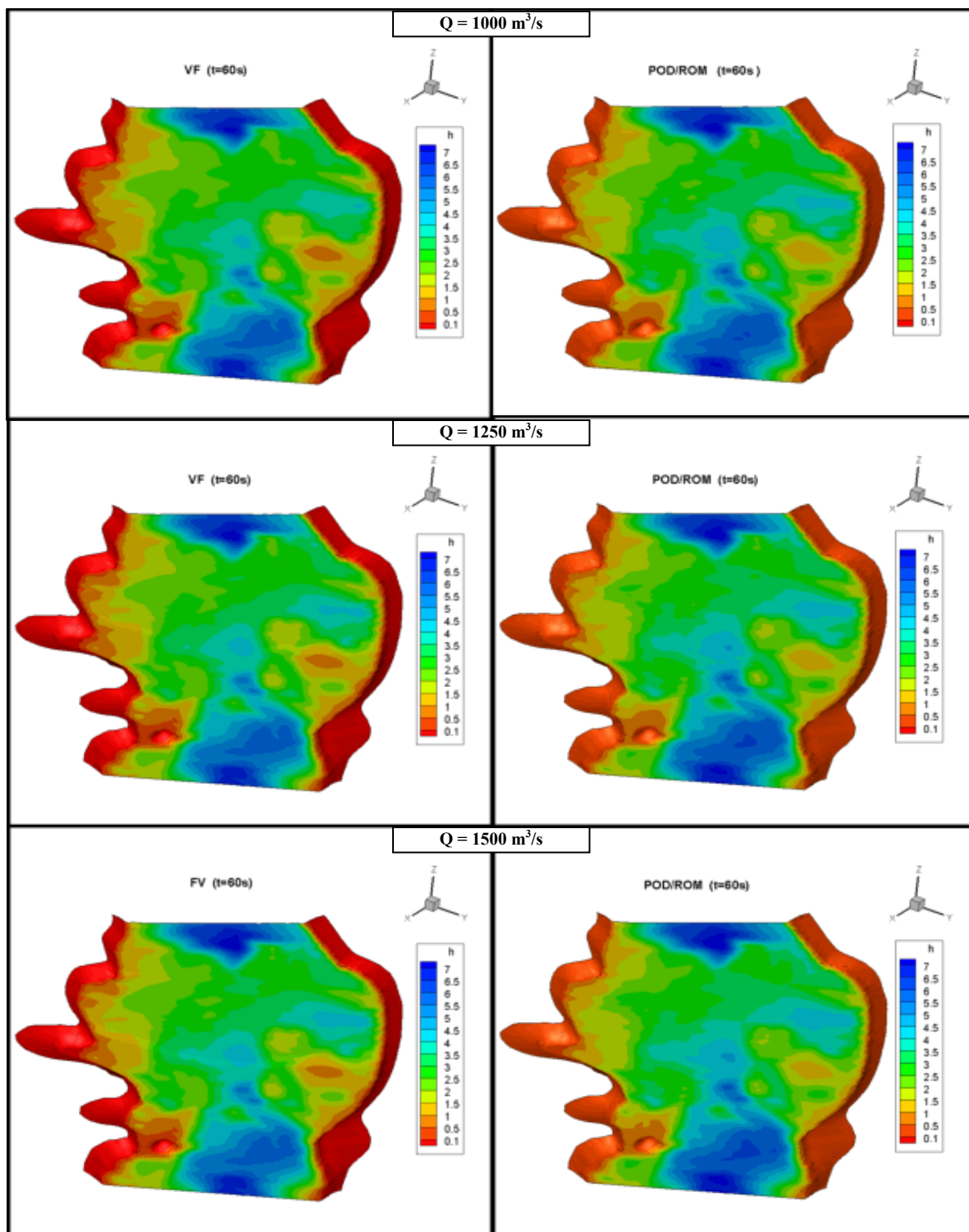
Figure 7.17 Estacade de Bordeaux Analyse de la sensibilité du POD/ROM à la variation du débit Contours de la hauteur d'eau comparés à l'instant t = 60 \text{ s}
