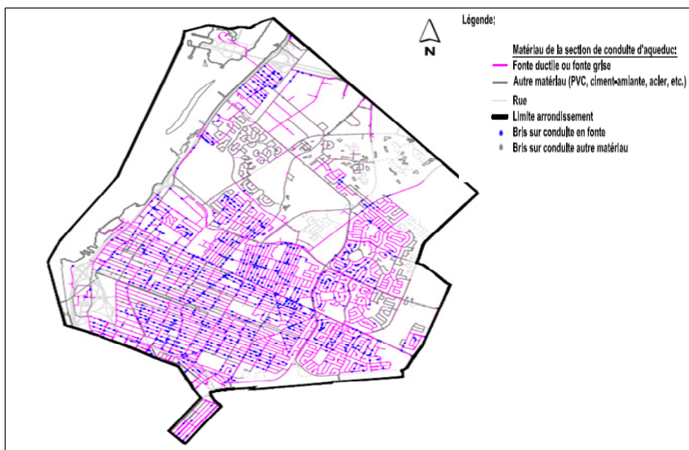
Figure FI - 1 Corrélation: matériaux de conduites – bris; Arrondissement AR-G.
