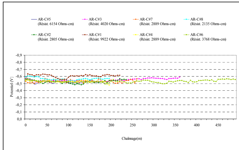
Figure 5.40 Potentiel statistique des conduites dans l'arrondissement AR-C.
