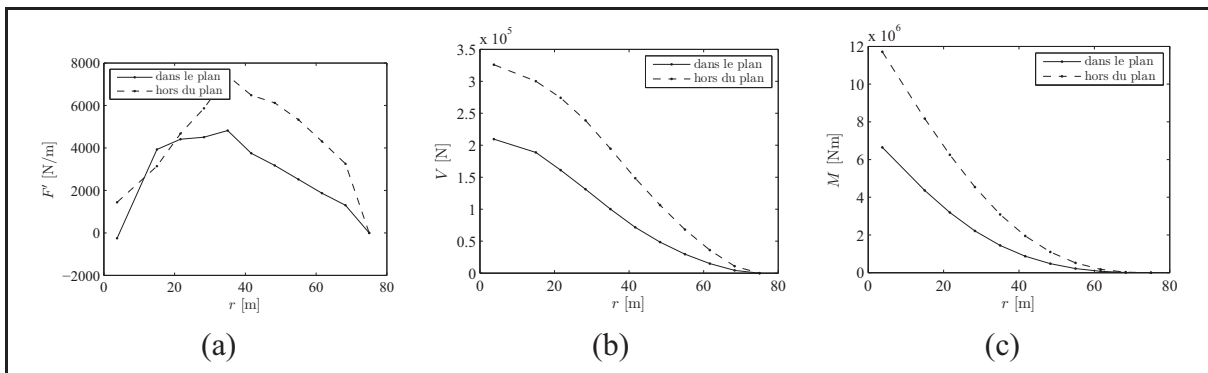
Figure 4.5 Chargements aérodynamiques pour le cas de chargement 2 (cisaillement horizontal, pale à l'horizontale, vitesse de vent de coupure). (a) Charges appliquées ( F' ). (b) Efforts tranchants ( V ). (c) Moments fléchissants ( M ).
