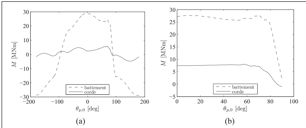
Figure 4.3 Moments fléchissants à l'emplacement pour une pale soumise au modèle de vent extrême. (a) Pale à la verticale. (b) Pale à l'horizontale (charges gravitationnelles incluses).
