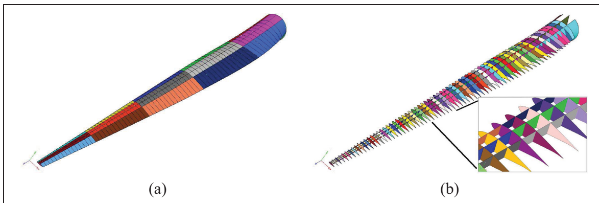
Figure 8.1 Modèle éléments finis de la pale pour l'optimisation dimensionnelle. (a) Semelles de longeron et coques. (b) Âmes et nervures.
