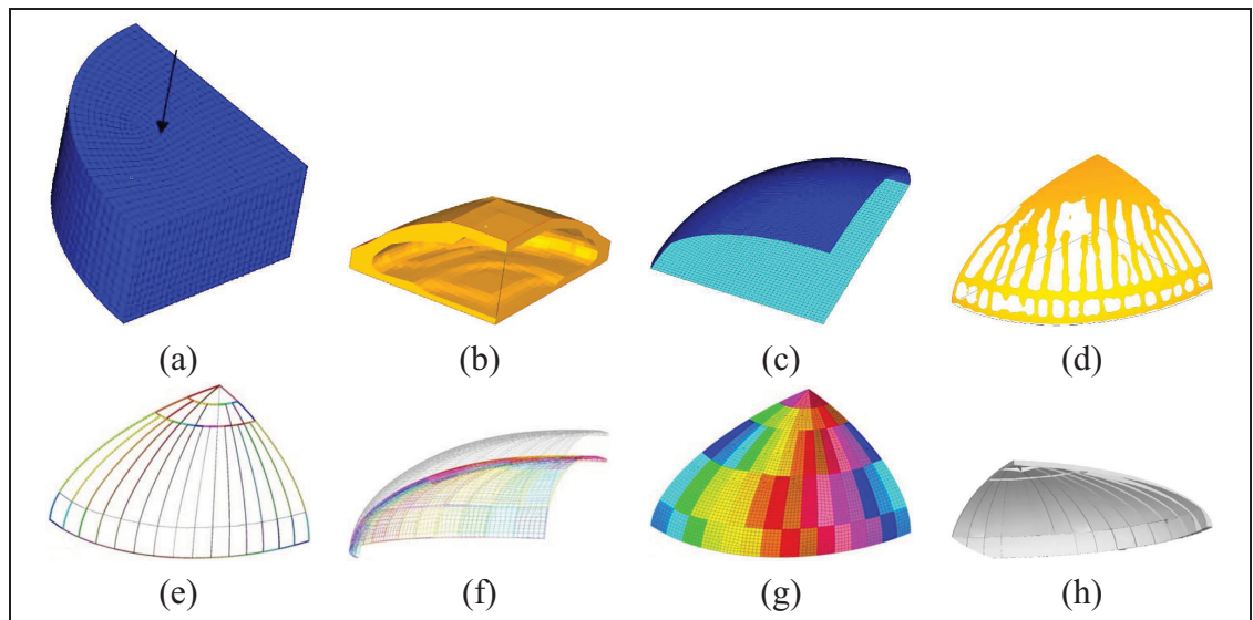
Figure 6.3 Exemple de processus d'optimisation. Adapté de Schramm et coll. (2004)
