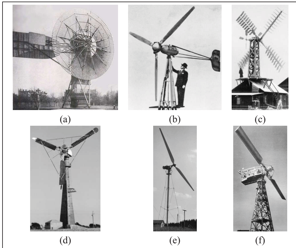
Figure 1.2 Éoliennes servant à la production d'électricité. (a) Éolienne de Charles F. Brush. (b) Éolienne de Marcellus et Joseph Jacobs. (c) Éolienne de Poul La Cour. (d) Éolienne de Johannes Juul (éolienne de Gedser). (e) Éolienne de Hütter. (f) Éolienne Putnam-Smith.
