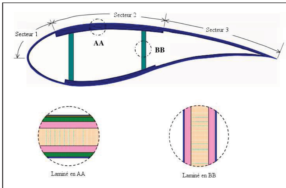
Figure 5.5 Section de pale de référence pour le code PRECOMP. Adapté de Bir (2005)
