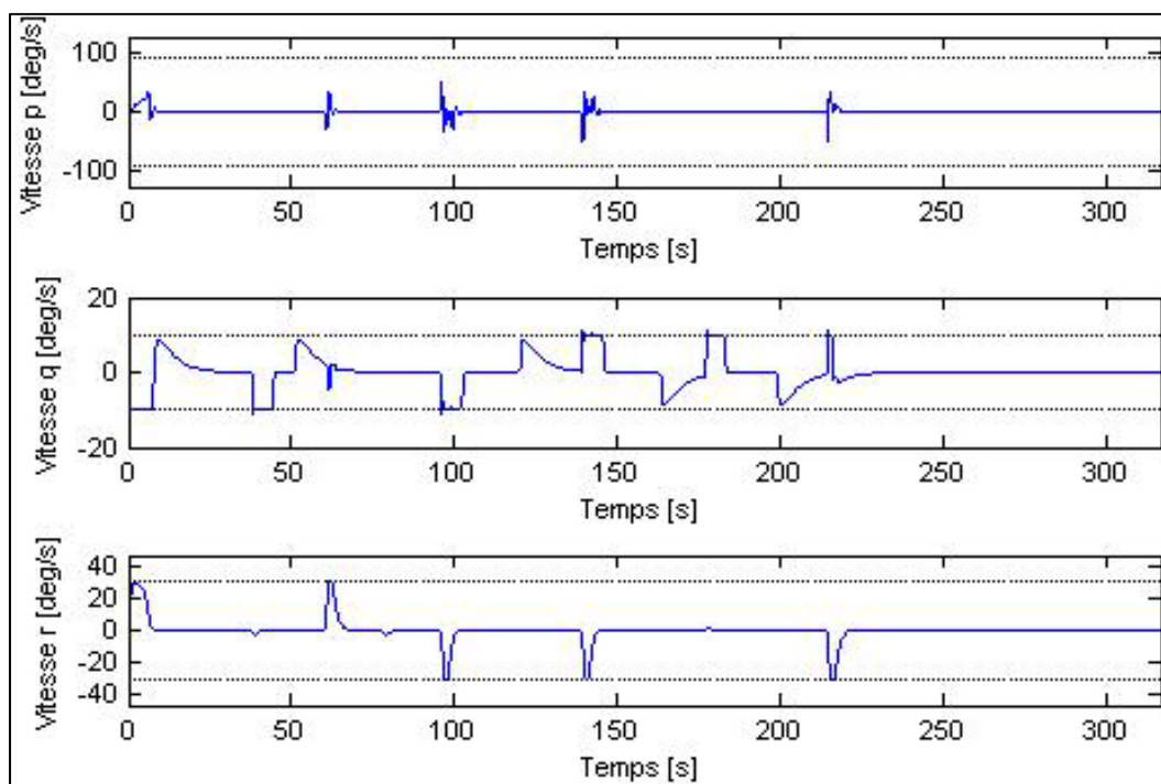
Figure 4.13 Évolution en fonction du temps de la vitesse de roulis p (deg/s), de la vitesse de tangage q (deg/s) et de la vitesse de lacet r (deg/s) pour une vitesse de consigne de 1 m/s.
