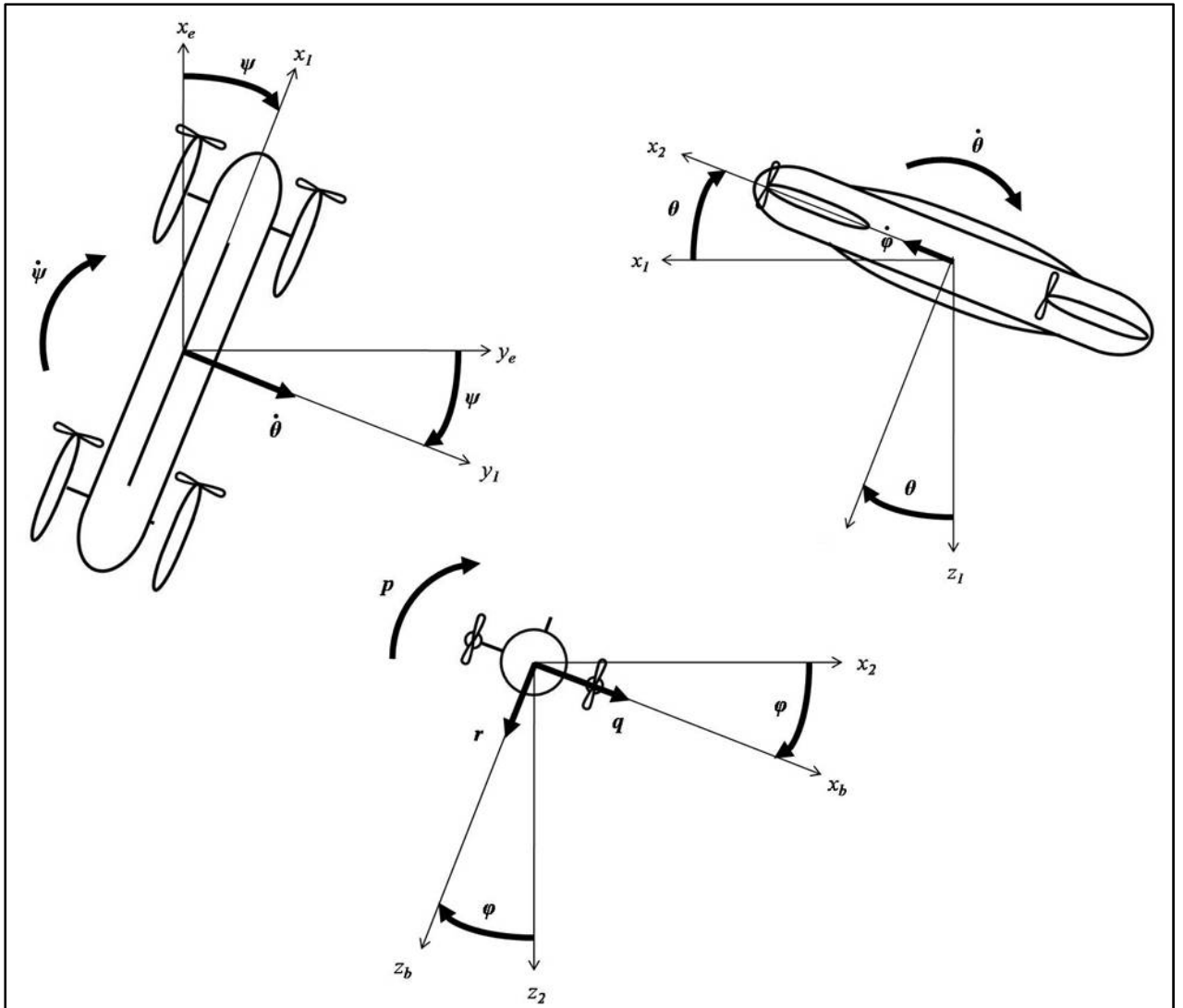
Figure 2.12 Séquences de rotation entre le repère « Earth » et le repère « Body ».
