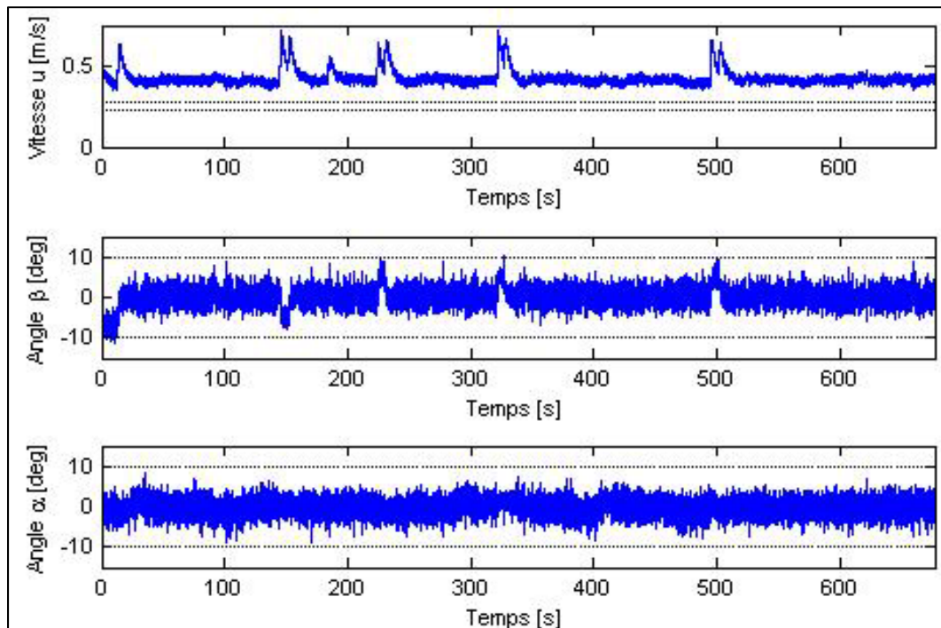
Figure 4.21 Évolution en fonction du temps de la vitesse d'avancement u (m/s), de l'angle d'attaque \alpha (deg) et de l'angle de dérapage \beta (deg) pour une vitesse de consigne de 0.25 m/s (avec du bruit de mesures).
