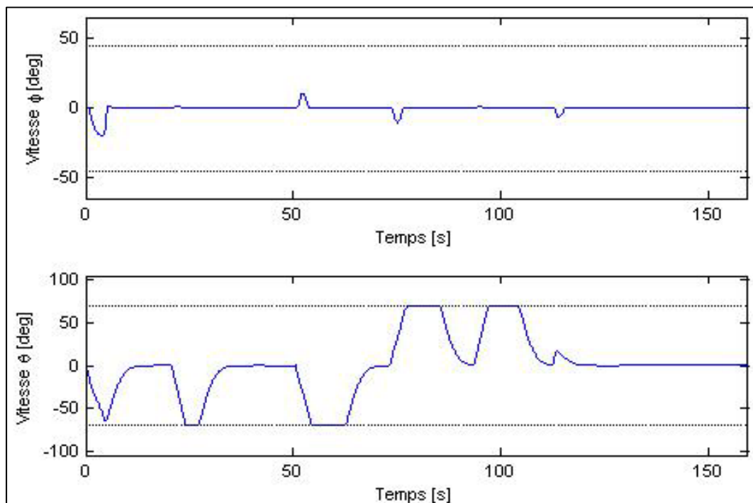
Figure 4.17 Évolution en fonction du temps de l'angle de gîte \phi (deg), de l'angle d'assiette \theta (deg) pour une vitesse de consigne de 2 m/s.
