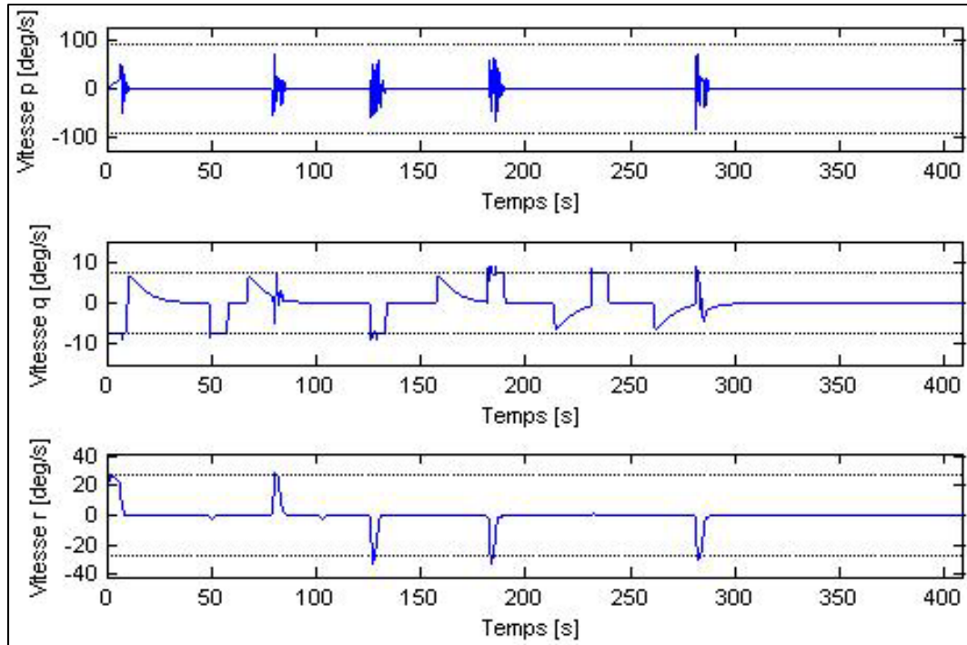
Figure 4.10 Évolution en fonction du temps de la vitesse de roulis p (deg/s), de la vitesse de tangage q (deg/s) et de la vitesse de lacet r (deg/s) pour une vitesse de consigne de 0.75 m/s.
