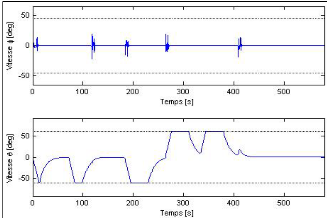
Figure 4.8 Évolution en fonction du temps de l'angle de gîte \phi (deg), de l'angle d'assiette \theta (deg) pour une vitesse de consigne de 0.5 m/s.
