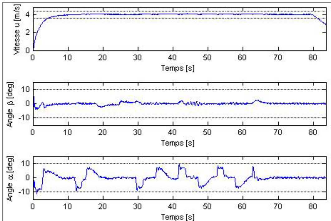
Figure 4.36 Évolution en fonction du temps de la vitesse d'avancement u (m/s), de l'angle d'attaque \alpha (deg) et de l'angle de dérapage \beta (deg) pour une vitesse de consigne de 4 m/s (avec du bruit de mesures).
