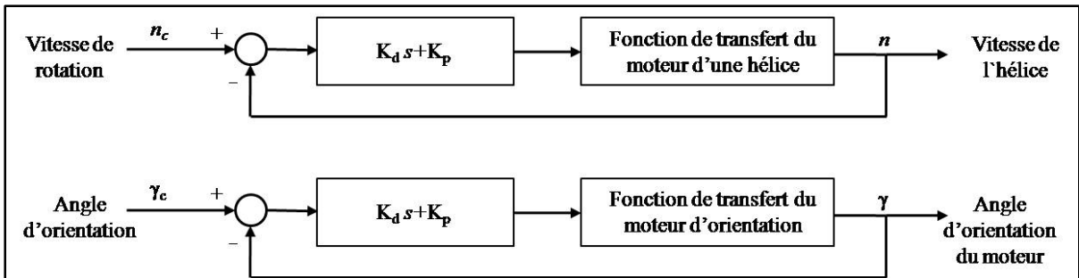
Figure 3.4 Schéma de la boucle de contrôle interne des moteurs d'hélices et des moteurs d'orientation.
