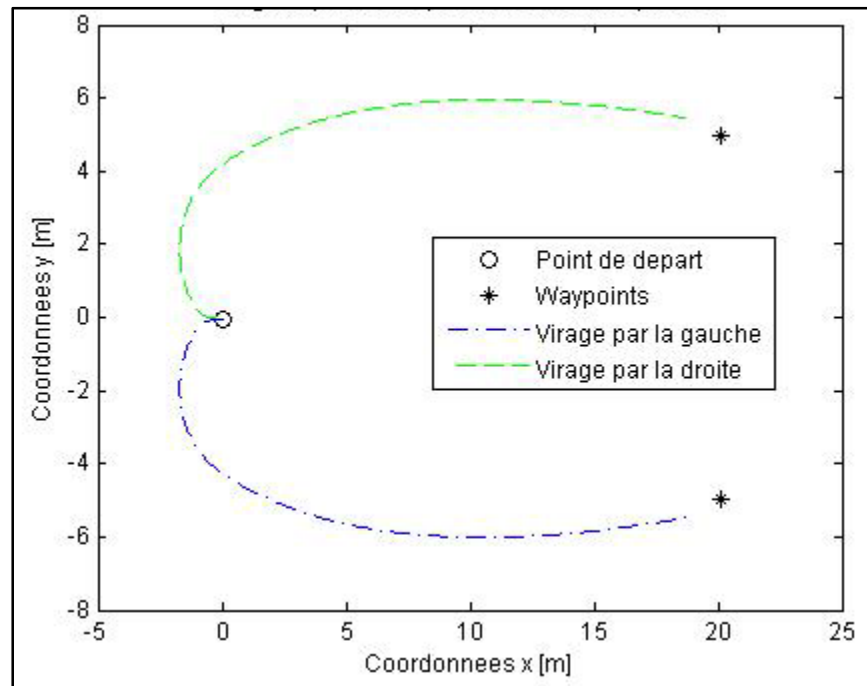
Figure 4.2 .Illustration du changement de cap suivant la position du waypoint à atteindre.
