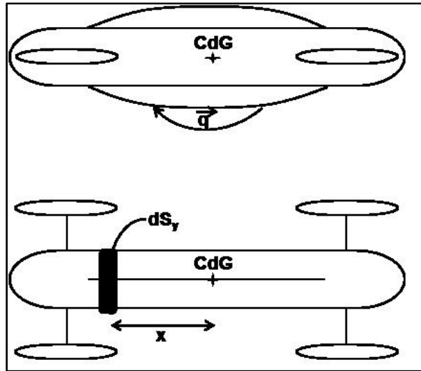
Figure 2.7 Schéma de l'amortissement quadratique de tangage.
