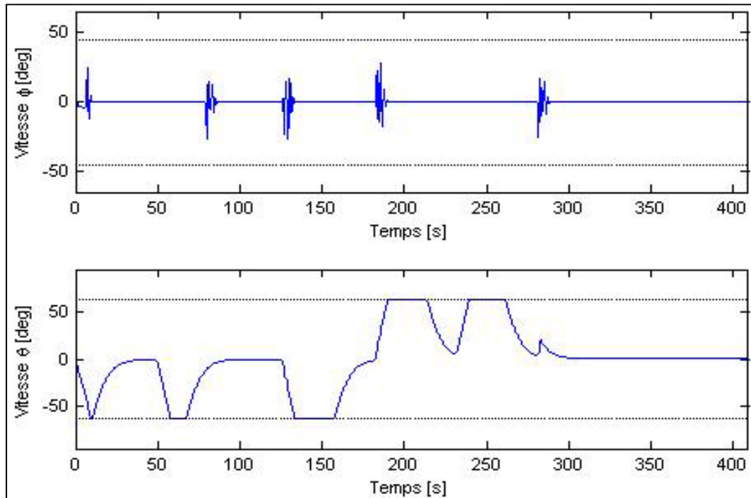
Figure 4.11 Évolution en fonction du temps de l'angle de gîte \phi (deg), de l'angle d'assiette \theta (deg) pour une vitesse de consigne de 0.75 m/s.
