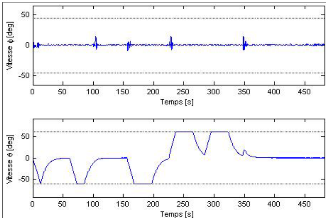
Figure 4.26 Évolution en fonction du temps de l'angle de gîte \phi (deg), de l'angle d'assiette \theta (deg) pour une vitesse de consigne de 0.5 m/s (avec du bruit de mesures).
