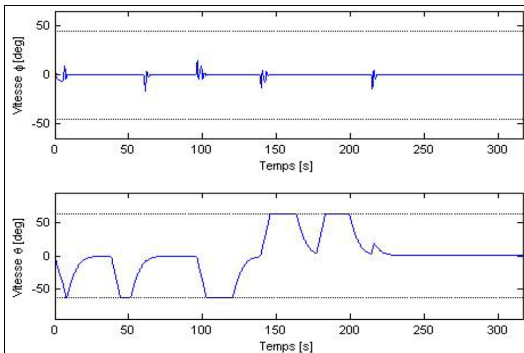
Figure 4.14 Évolution en fonction du temps de l'angle de gîte \phi (deg), de l'angle d'assiette \theta (deg) pour une vitesse de consigne de 1 m/s.
