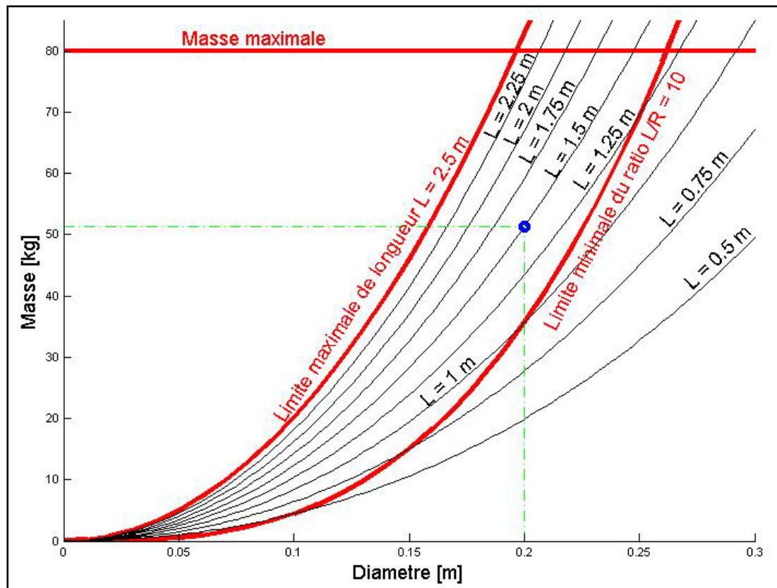
Figure 1.4 Graphique de dimensionnement extérieur du drone.
