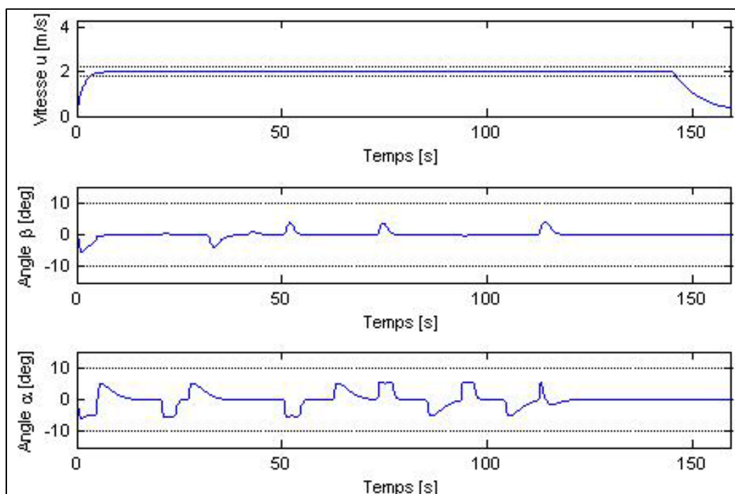
Figure 4.15 Évolution en fonction du temps de la vitesse d'avancement u (m/s), de l'angle d'attaque \alpha (deg) et de l'angle de dérapage \beta (deg) pour une vitesse de consigne de 2 m/s.
