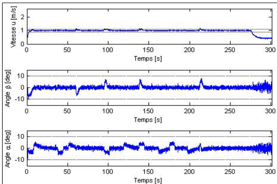
Figure 4.30 Évolution en fonction du temps de la vitesse d'avancement u (m/s), de l'angle d'attaque \alpha (deg) et de l'angle de dérapage \beta (deg) pour une vitesse de consigne de 1 m/s (avec du bruit de mesures).
