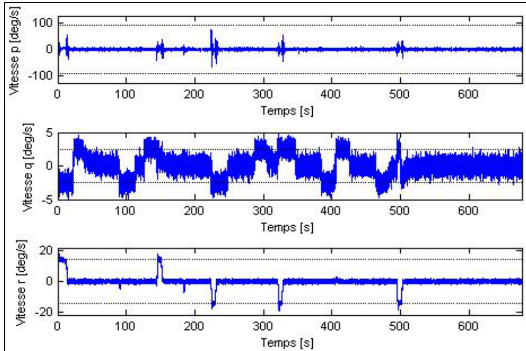
Figure 4.22 Évolution en fonction du temps de la vitesse de roulis p (deg/s), de la vitesse de tangage q (deg/s) et de la vitesse de lacet r (deg/s) pour une vitesse de consigne de 0.25 m/s (avec du bruit de mesures).
