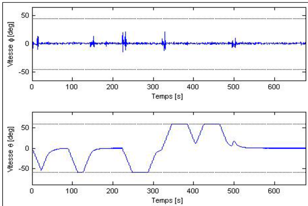
Figure 4.23 Évolution en fonction du temps de l'angle de gîte \phi (deg), de l'angle d'assiette \theta (deg) pour une vitesse de consigne de 0.25 m/s (avec du bruit de mesures).
