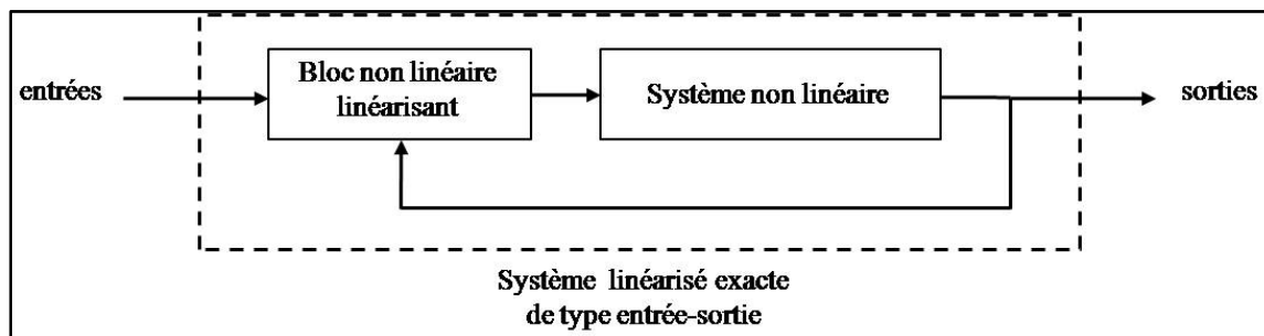
Figure 3.1 Schéma de la méthode de linéarisation exacte entrées-sorties.
