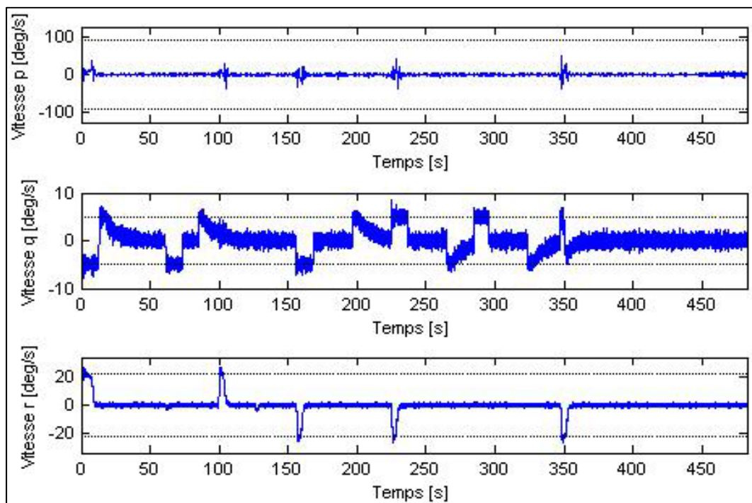
Figure 4.25 Évolution en fonction du temps de la vitesse de roulis p (deg/s), de la vitesse de tangage q (deg/s) et de la vitesse de lacet r (deg/s) pour une vitesse de consigne de 0.5 m/s (avec du bruit de mesures).
