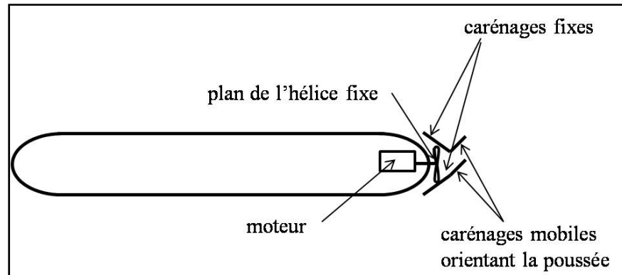
Figure 1.6 Schéma de principe de la poussée vectorielle par déviation du jet.
