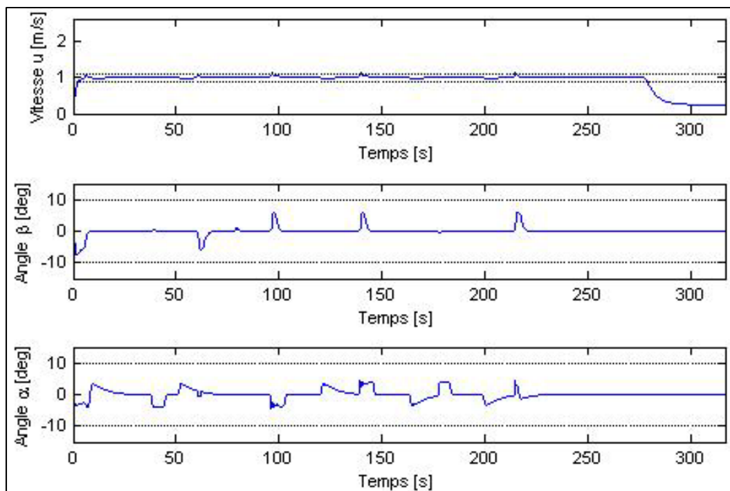
Figure 4.12 Évolution en fonction du temps de la vitesse d'avancement u (m/s), de l'angle d'attaque \alpha (deg) et de l'angle de dérapage \beta (deg) pour une vitesse de consigne de 1 m/s.
