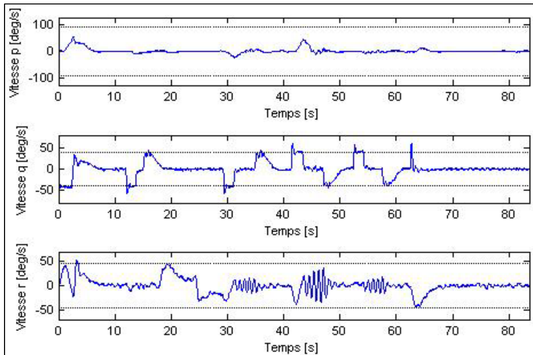
Figure 4.37 Évolution en fonction du temps de la vitesse de roulis p (deg/s), de la vitesse de tangage q (deg/s) et de la vitesse de lacet r (deg/s) pour une vitesse de consigne de 4 m/s (avec du bruit de mesures).
