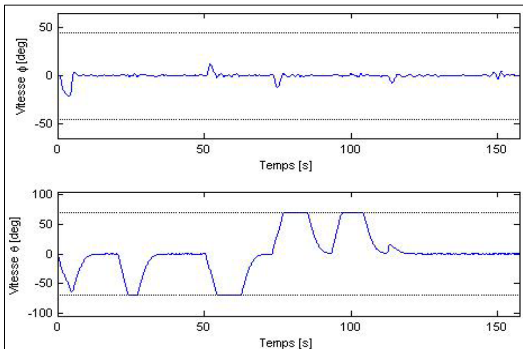
Figure 4.35 Évolution en fonction du temps de l'angle de gîte \phi (deg), de l'angle d'assiette \theta (deg) pour une vitesse de consigne de 2 m/s (avec du bruit de mesures).
