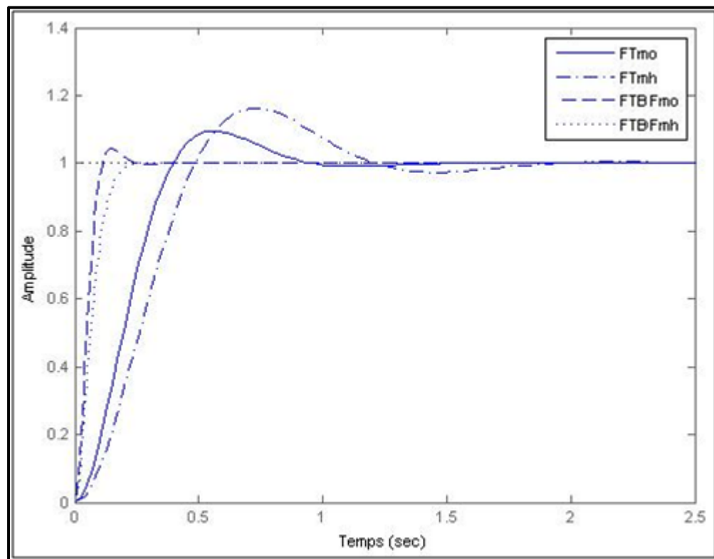
Figure 3.5 Réponses temporelles naturelles (FT) et forcées (FTBF) des moteurs d'orientation et des moteurs d'hélice.
