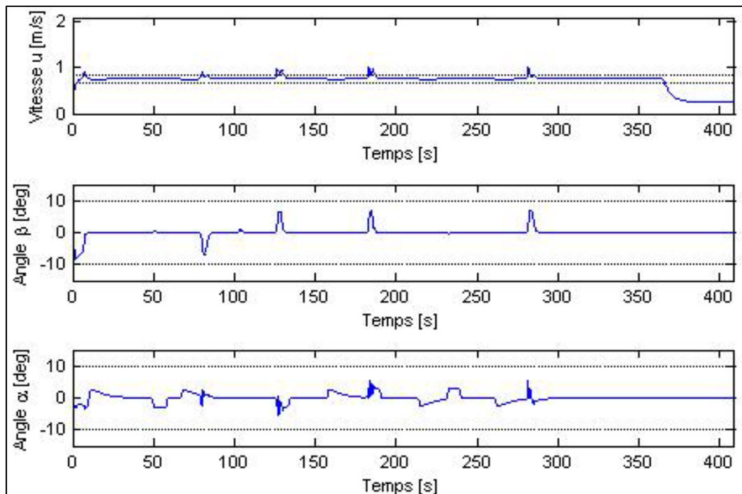
Figure 4.9 Évolution en fonction du temps de la vitesse d'avancement u (m/s), de l'angle d'attaque \alpha (deg) et de l'angle de dérapage \beta (deg) pour une vitesse de consigne de 0.75 m/s.
