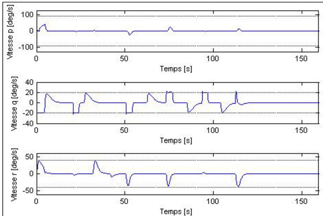
Figure 4.16 Évolution en fonction du temps de la vitesse de roulis p (deg/s), de la vitesse de tangage q (deg/s) et de la vitesse de lacet r (deg/s) pour une vitesse de consigne de 2 m/s.
