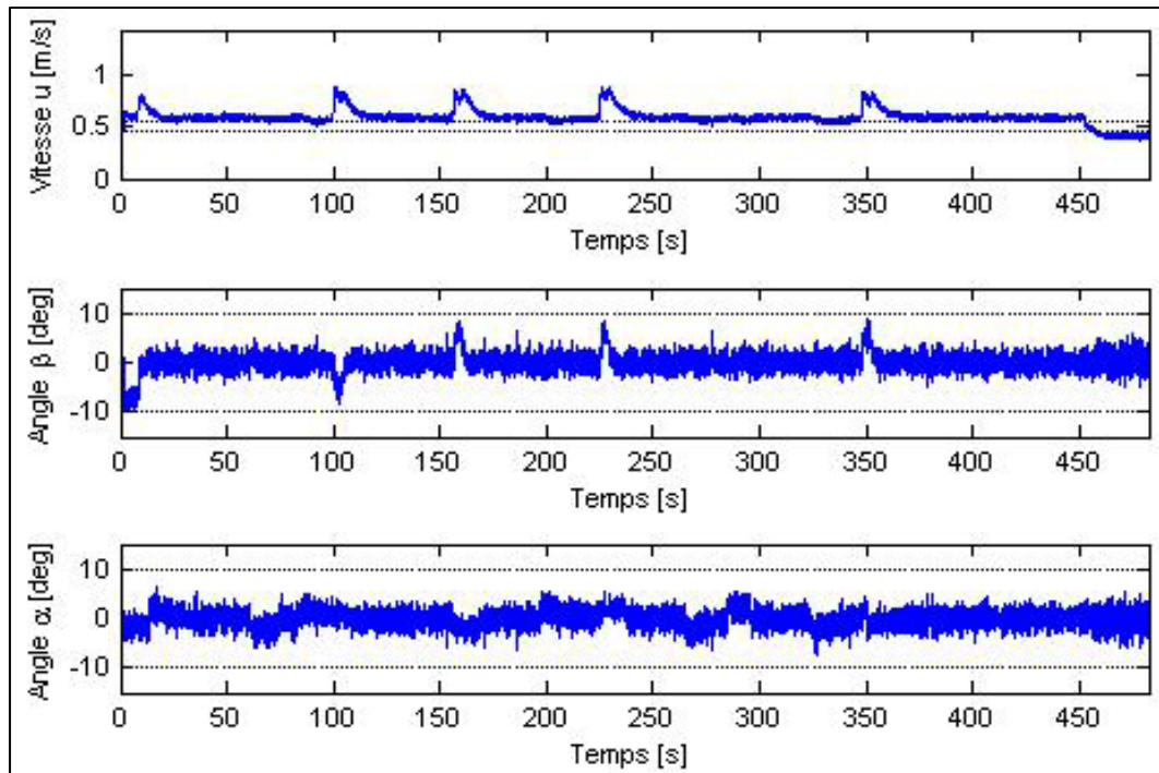
Figure 4.24 Évolution en fonction du temps de la vitesse d'avancement u (m/s), de l'angle d'attaque \alpha (deg) et de l'angle de dérapage \beta (deg) pour une vitesse de consigne de 0.5 m/s (avec du bruit de mesures).
