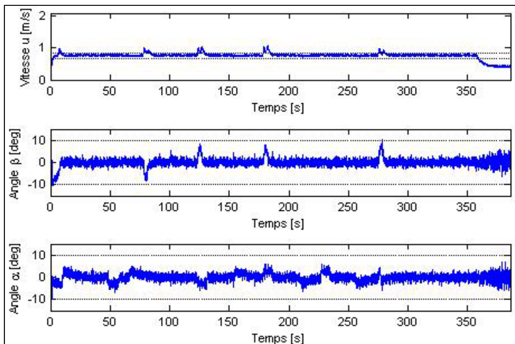
Figure 4.27 Évolution en fonction du temps de la vitesse d'avancement u (m/s), de l'angle d'attaque \alpha (deg) et de l'angle de dérapage \beta (deg) pour une vitesse de consigne de 0.75 m/s (avec du bruit de mesures).
