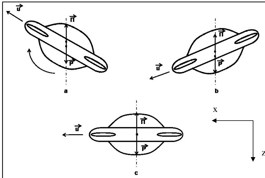
Figure 2.11 Différentes situations d'équilibre statique. a) Centre de gravité situé au dessus du centre de poussée, b) Centrage avant, c) Centrage idéal
