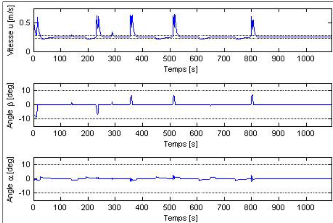
Figure 4.3 Évolution en fonction du temps de la vitesse d'avancement u (m/s), de l'angle d'attaque \alpha (deg) et de l'angle de dérapage \beta (deg) pour une vitesse de consigne de 0.25 m/s.
