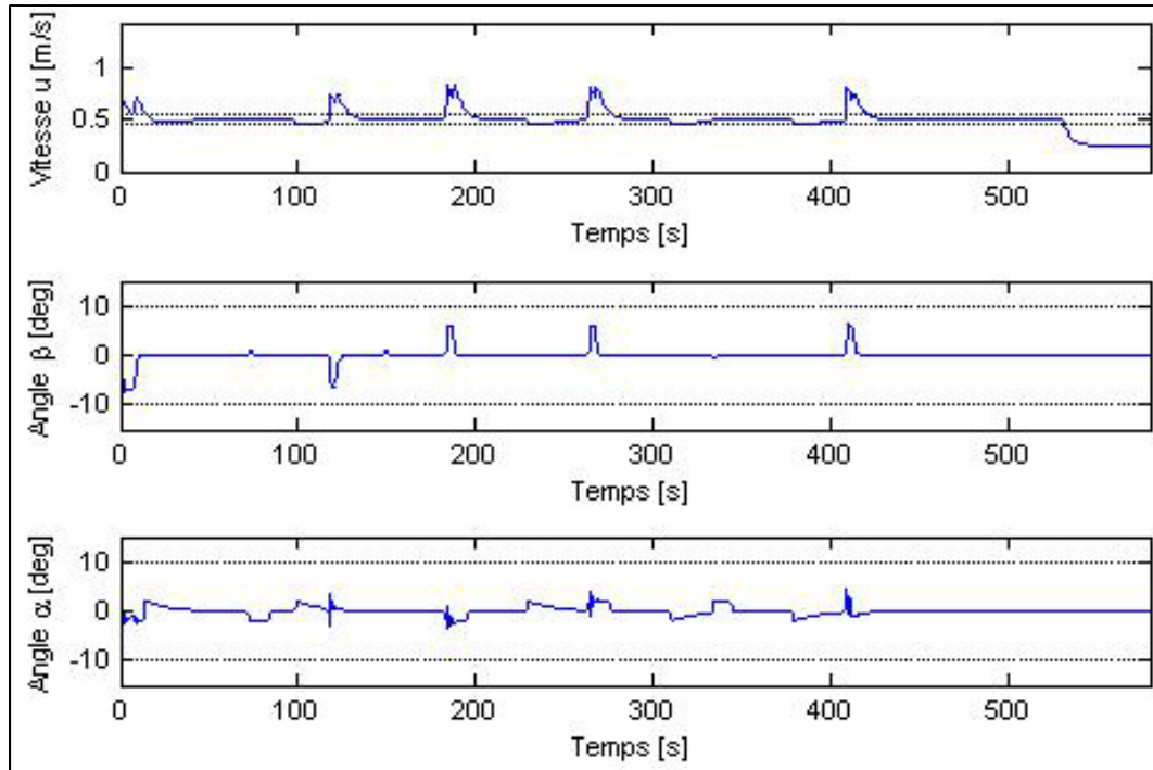
Figure 4.6 Évolution en fonction du temps de la vitesse d'avancement u (m/s), de l'angle d'attaque \alpha (deg) et de l'angle de dérapage \beta (deg) pour une vitesse de consigne de 0.5 m/s.
