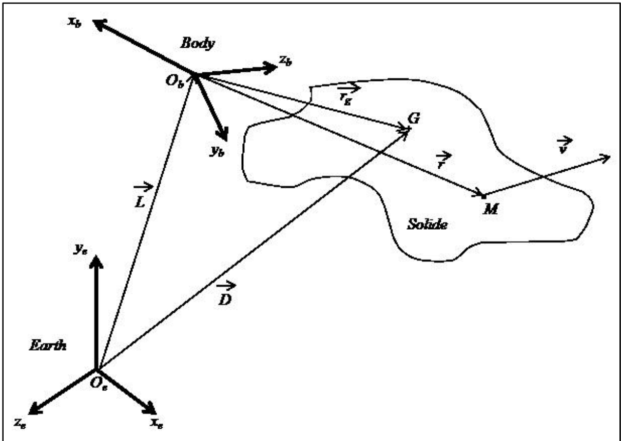
Figure 2.1 Schéma d'un solide indéformable lié à un repère terrestre et au repère lié au corps.
