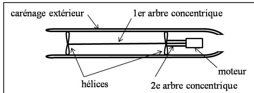
Figure 1.8 Concept de deux hélices contrarotatives dans un flux d'eau. (transmission par arbres concentriques)
