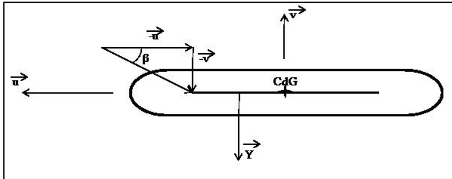
Figure 2.2 Schéma de la dérive latérale et de l'angle de dérapage.
