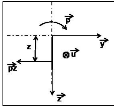
Figure 2.5 Vitesse linéaire d'un point distant de l'axe de roulis.
