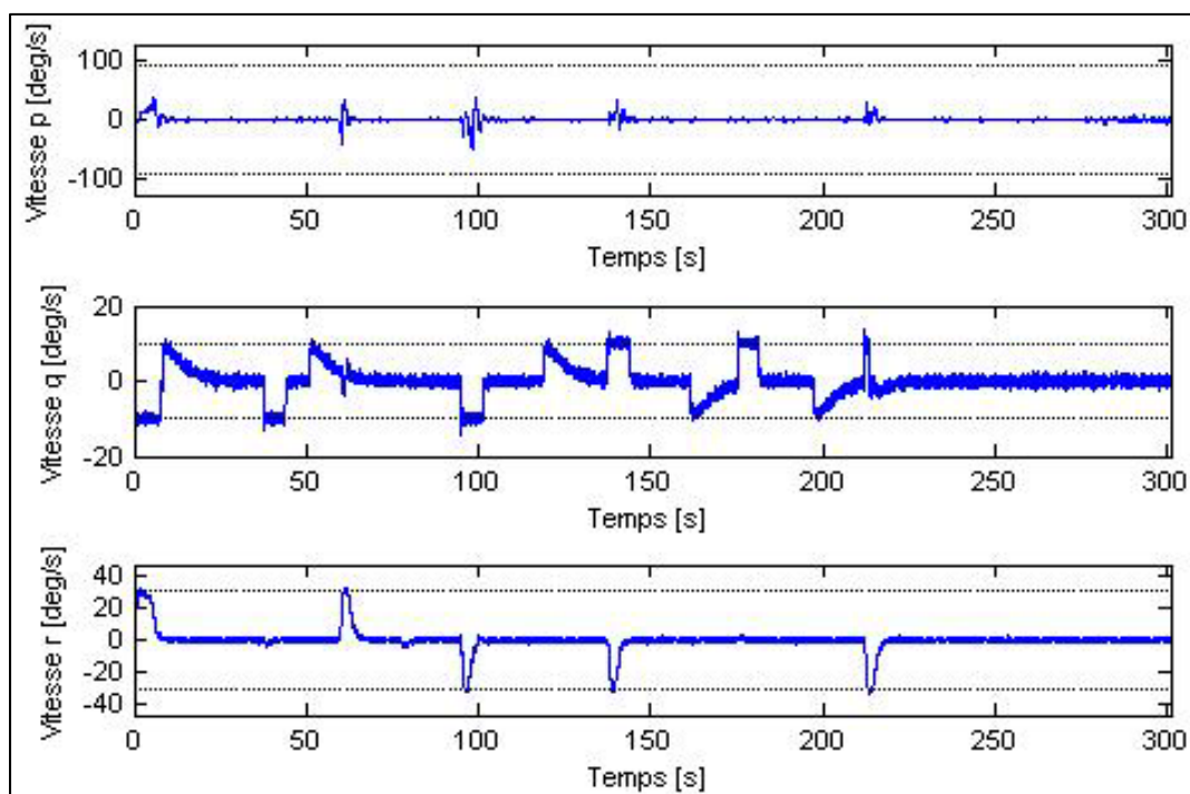
Figure 4.31 Évolution en fonction du temps de la vitesse de roulis p (deg/s), de la vitesse de tangage q (deg/s) et de la vitesse de lacet r (deg/s) pour une vitesse de consigne de 1 m/s (avec du bruit de mesures).
