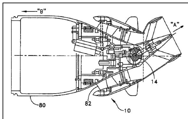
Figure 1.7 Plan détaillé de la tuyère orientable pour UUV. (extrait du brevet US 7 465 201)
