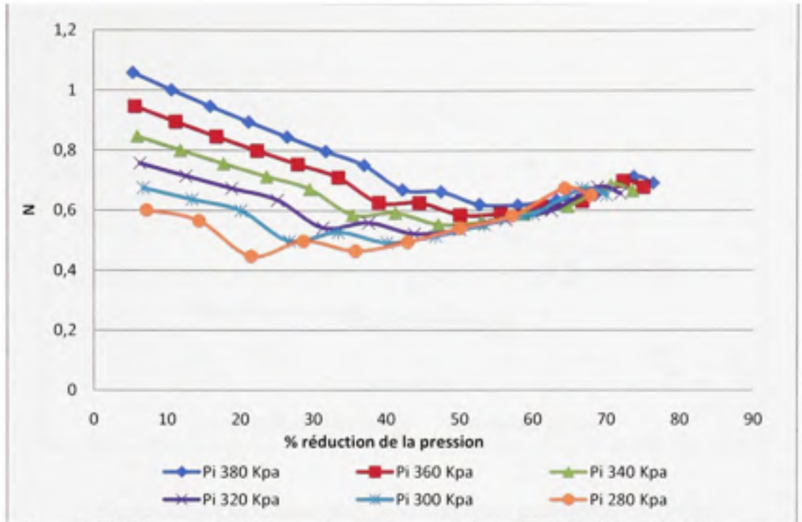
Figure 3.17 La variation de N en fonction de taux de réduction de fuite pou différentes pressions initiales – conduite très flexible.
