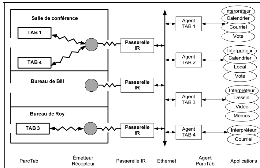
Figure 3.2 Architecture du ParcTab. Adaptée de want et al. (1995, p. 15)
