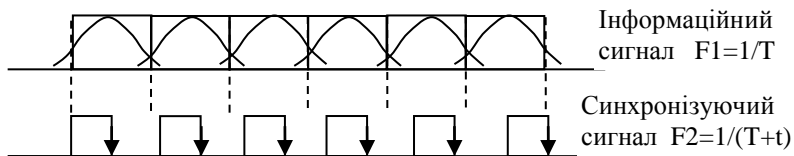
Рис. 7. Частота інформаційного сигналу і синхронізуючого сигналу не співпадають
