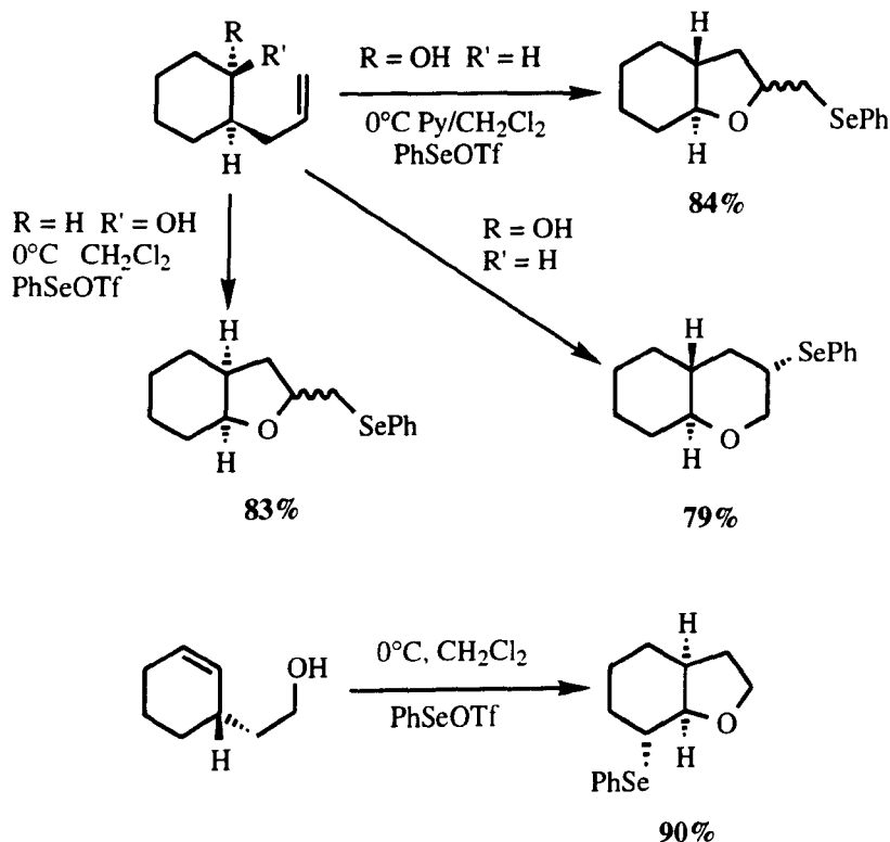
(Scheme 17)
