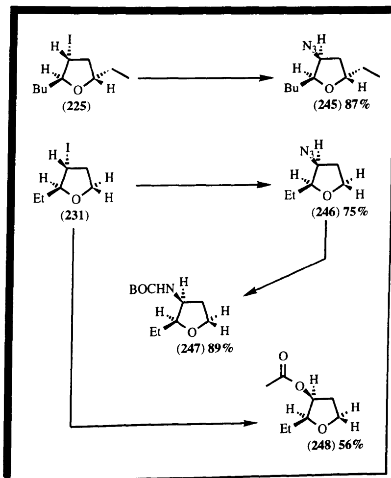
(Scheme 55)
