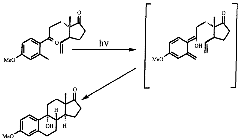
(Scheme 22)
