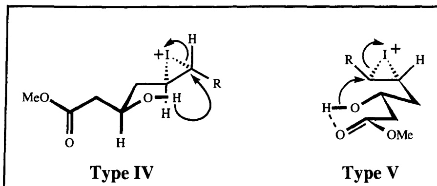
(Scheme 37)
