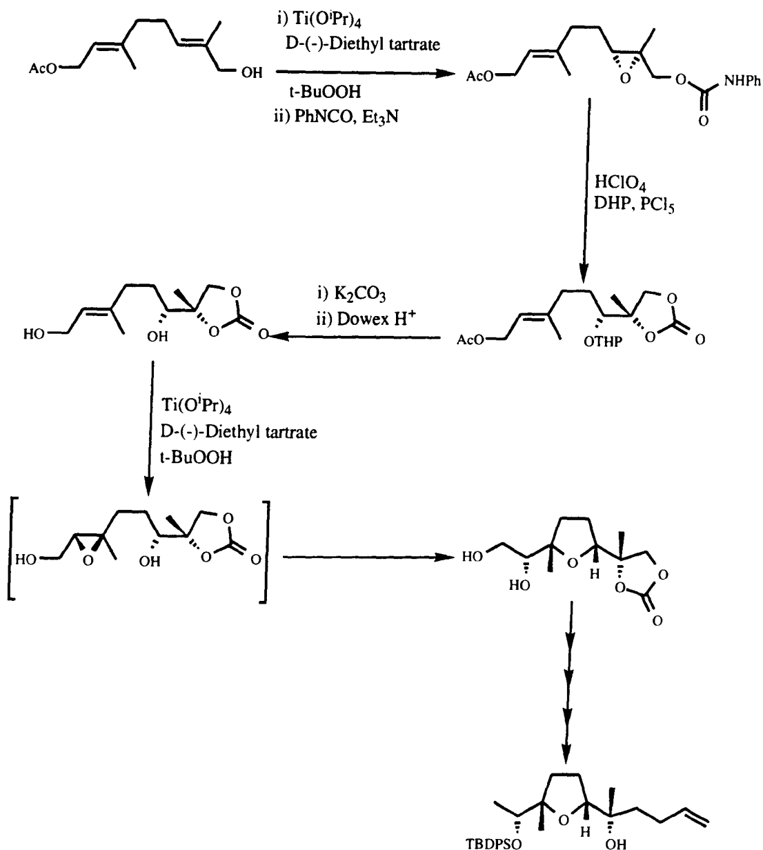
(Scheme 23)
