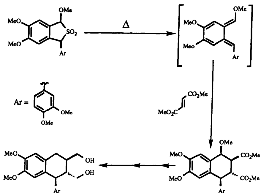
(Scheme 24)
