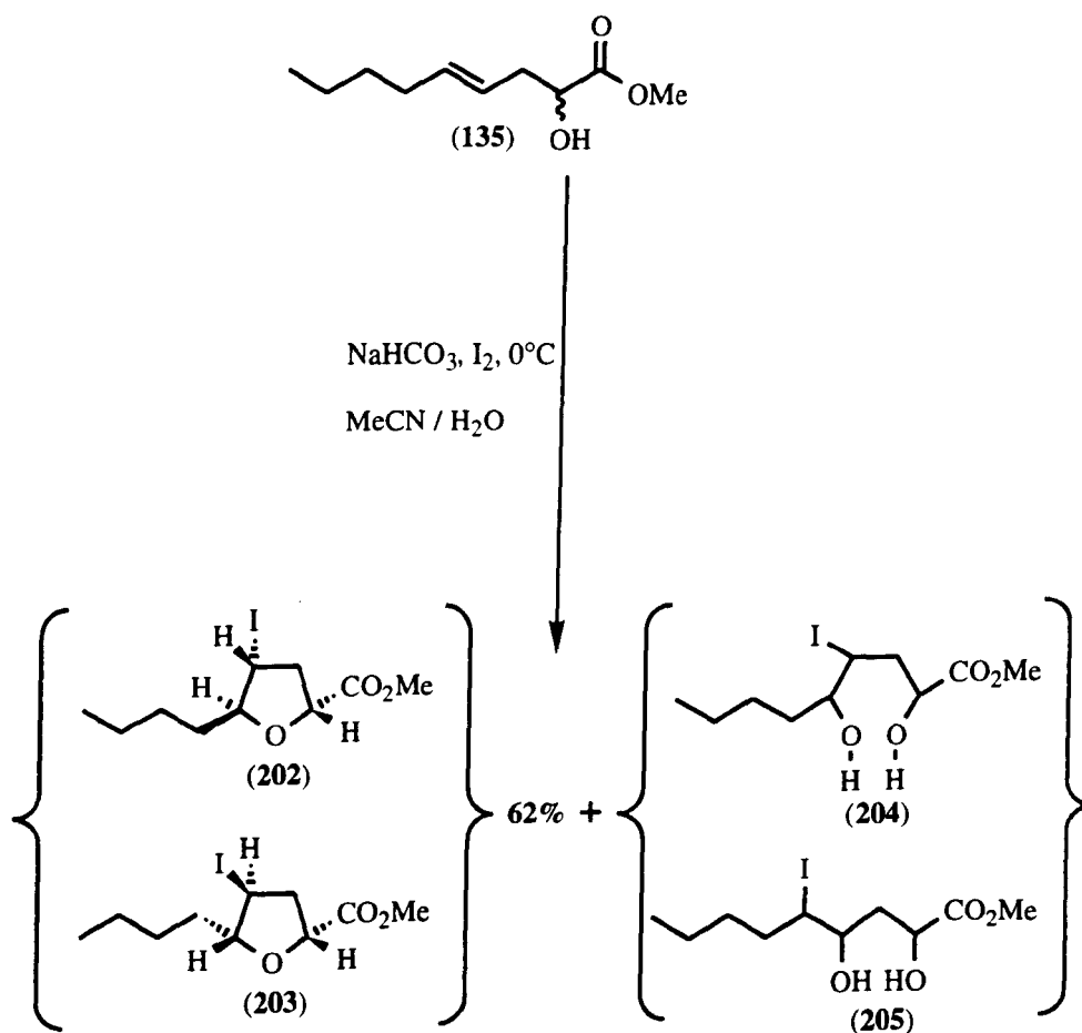
(Scheme 35)
