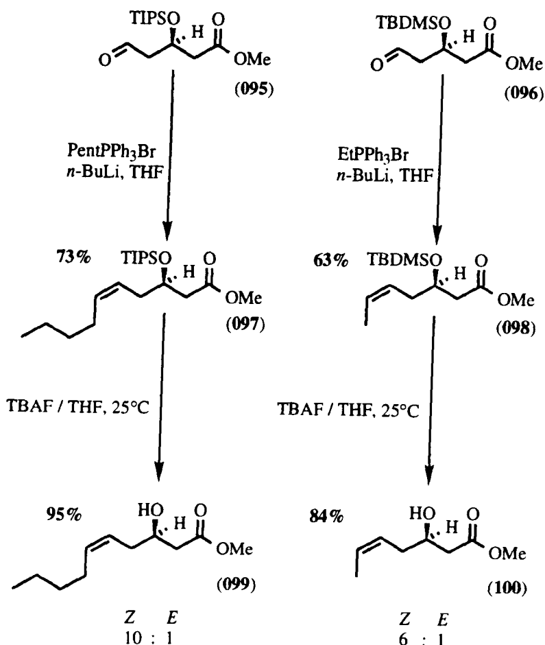
(Scheme 5)
