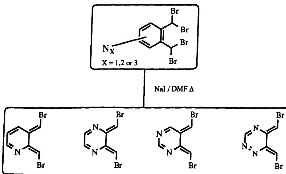
(Scheme 46)
