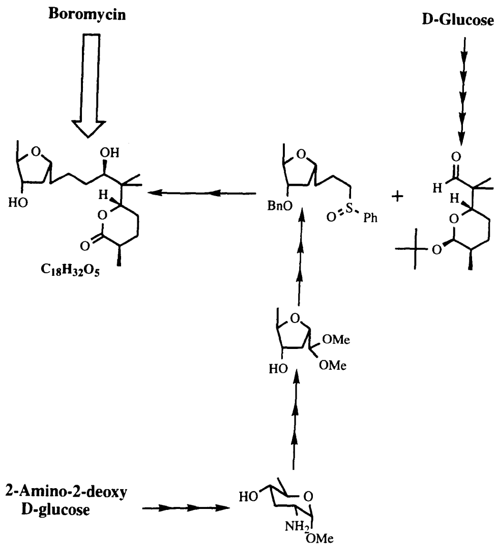
(Scheme 53)
