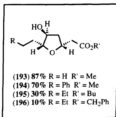
(Scheme 31)
