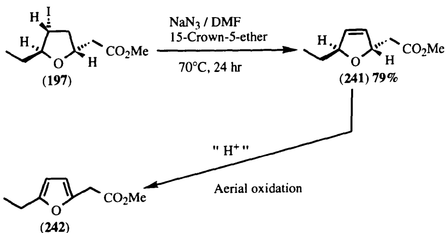
(Scheme 53)
