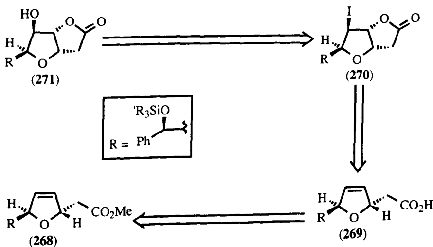
(Scheme 65)
