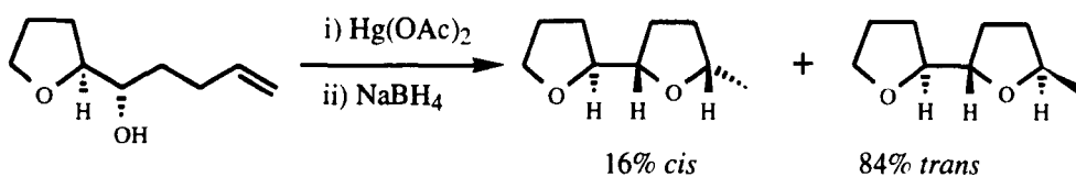
(Scheme 24)
