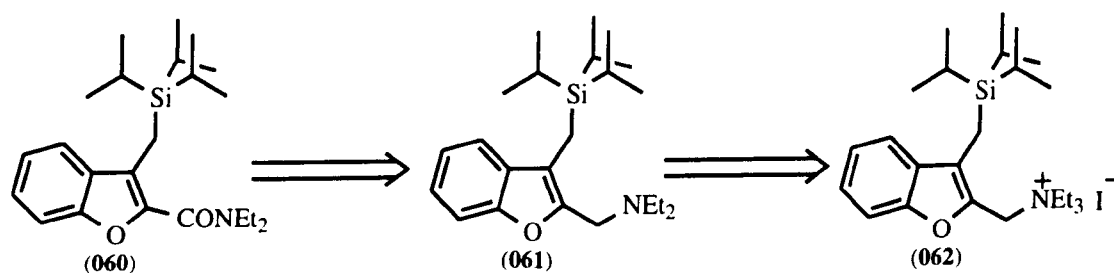
(Scheme 23)
