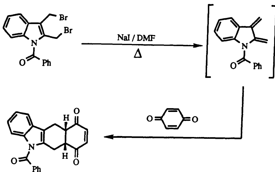
(Scheme 45)
