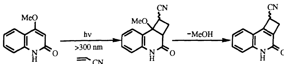
(Scheme 36)
