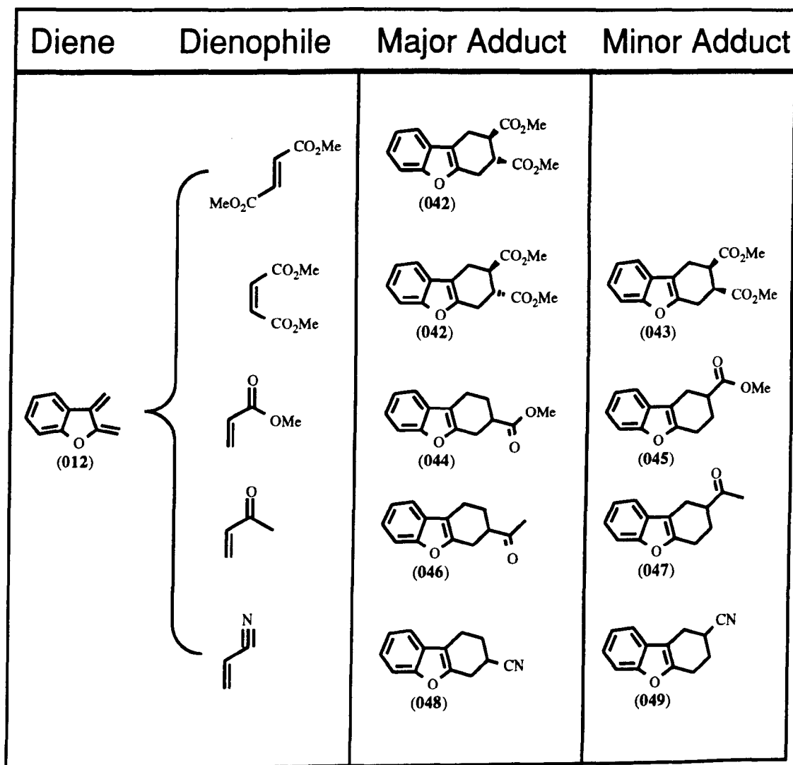
(Scheme 17)
