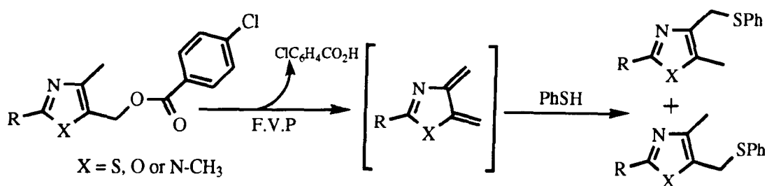
(Scheme 53)
