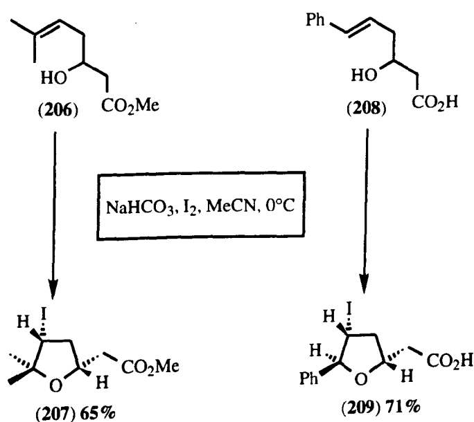
(Scheme 36)
