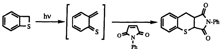
(Scheme 18)
