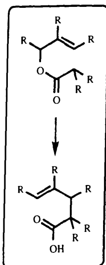
(Scheme 34)
