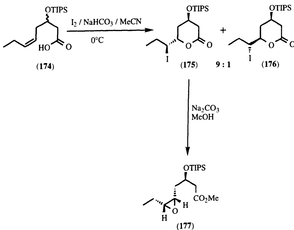
(Scheme 22)
