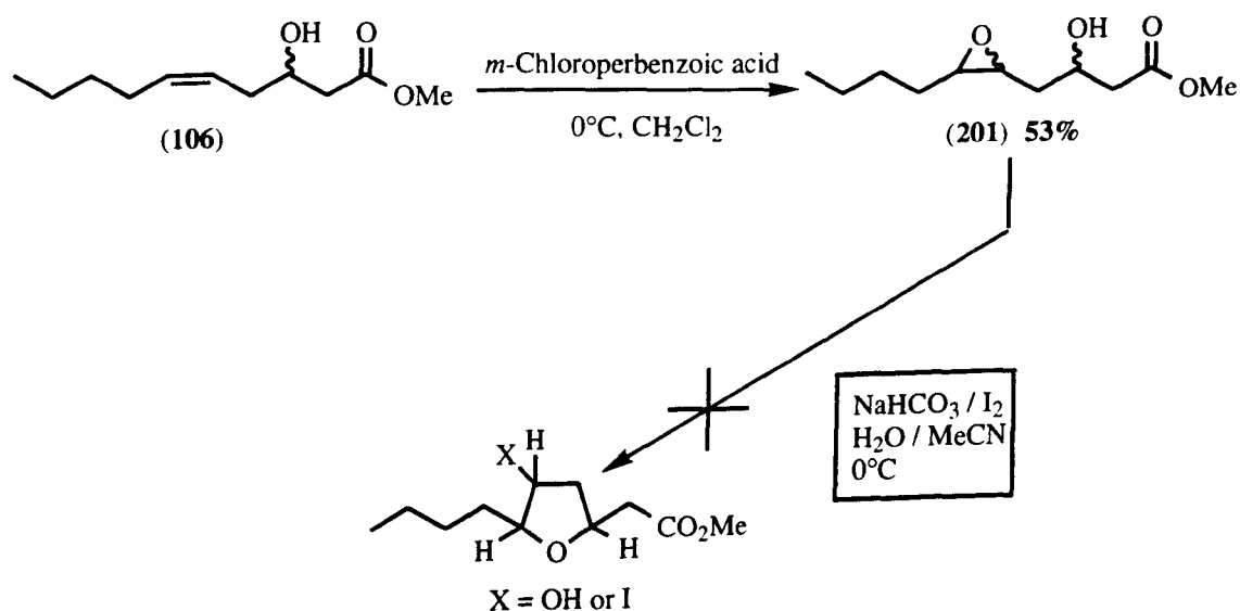
(Scheme 34)
