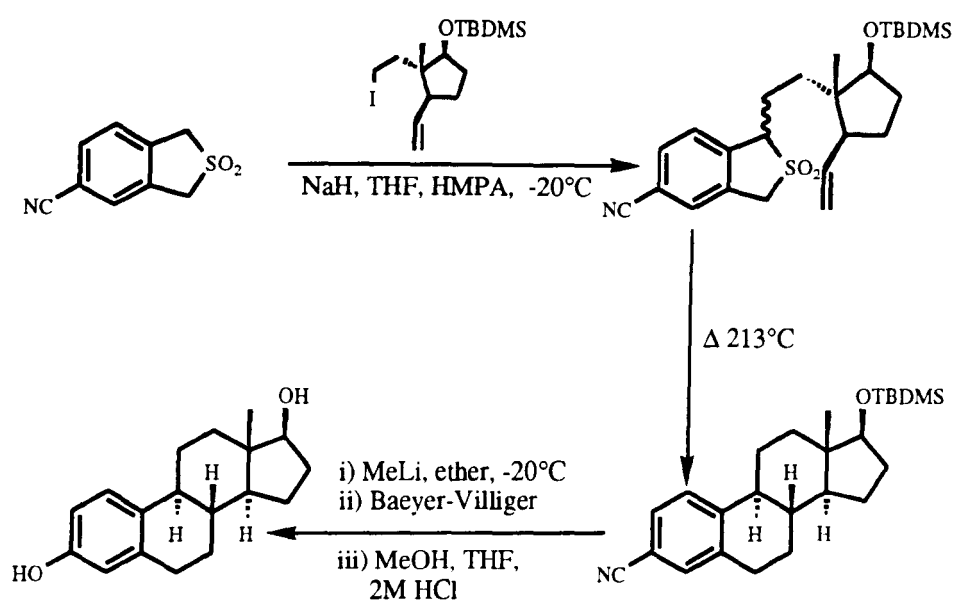
(Scheme 21)
