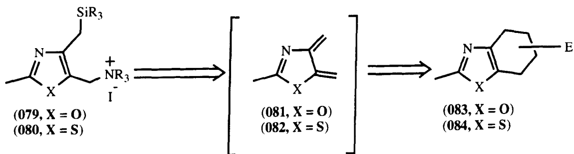
(Scheme 31)
