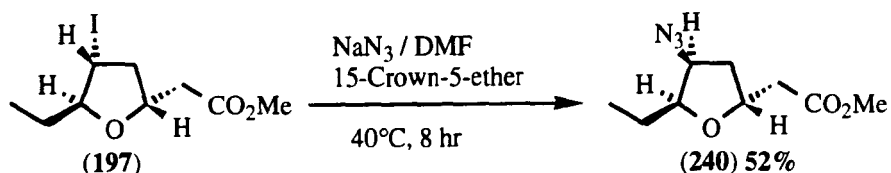
(Scheme 52)
