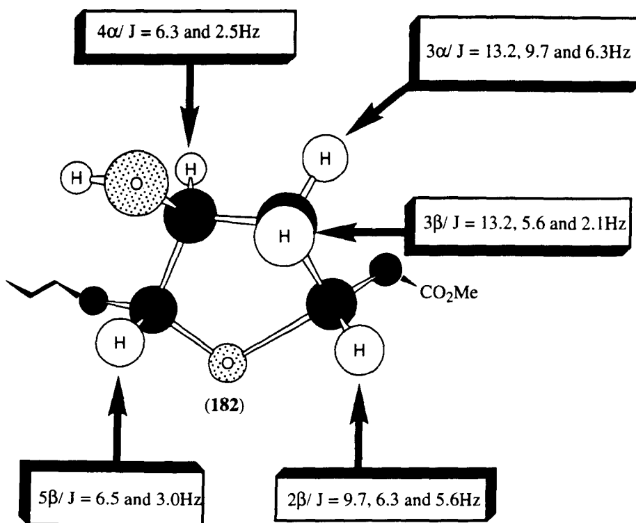
(Scheme 26)
