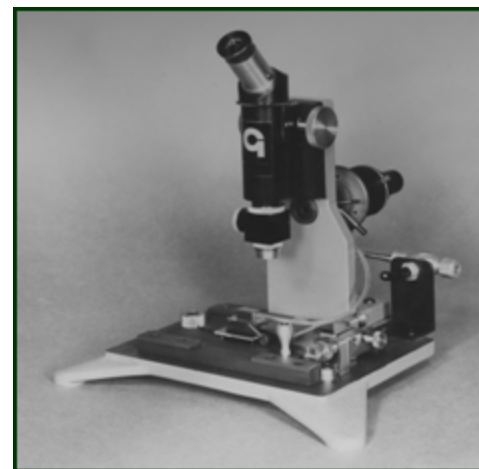
Микроскоп за центрирање првог умањења Mann 992A
