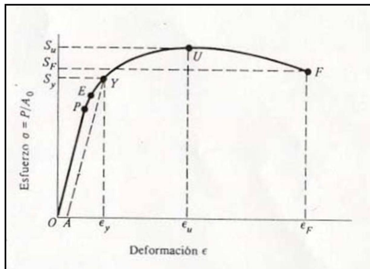
Fig. 2.4 Curva esfuerzo real-deformación real: Diagrama esfuerzo-deformación obtenido a partir del ensayo normal a la tensión de una manera dúctil. El punto P indica el límite de proporcionalidad; E, el límite elástico Y, la resistencia de fluencia convencional determinada por corrimiento paralelo (offset) según la deformación seleccionada OA; U; la resistencia última o máxima, y F, el esfuerzo de fractura o ruptura. Extraído de Collins et al
