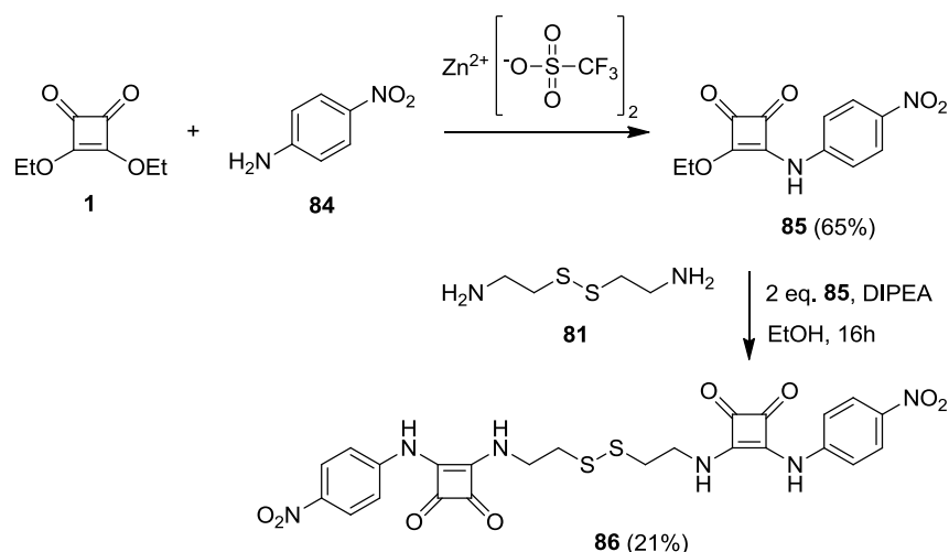
Esquema 67 – Síntesis del modelo autoinmoleto no fluorescente 86 .
