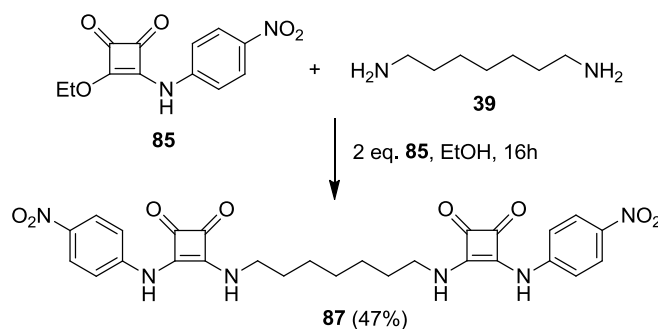
Esquema 68 – Síntesis del conjugado sin capacidad autoinmoleto 87 .
