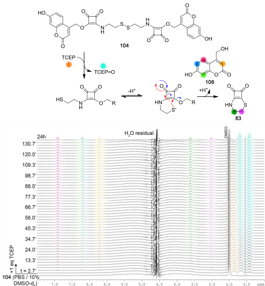
Figura 132 – Mecanismo propuesto de autoinmolación del compuesto 104 (1 mM) mediante reducción con TCEP, asignación de las señales características, y espectros de 1 H-RMN donde se ha señalado la evolución de las señales de la cumarina 106 , el ciclo C1NS 83 y la TCEP en su forma oxidada.
