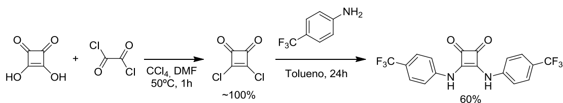
Esquema 2 – Síntesis de esquaramidas derivadas de aminas poco nucleófilas mediante el uso del dicloruro del ácido escuárico como intermedio. 7
