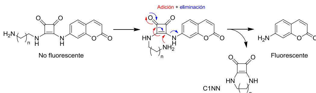
Esquema 62 – Evolución del espaciador autoinmolativo mediante la acción de aminas primarias sobre escuarlamidas derivadas de anilinas.
