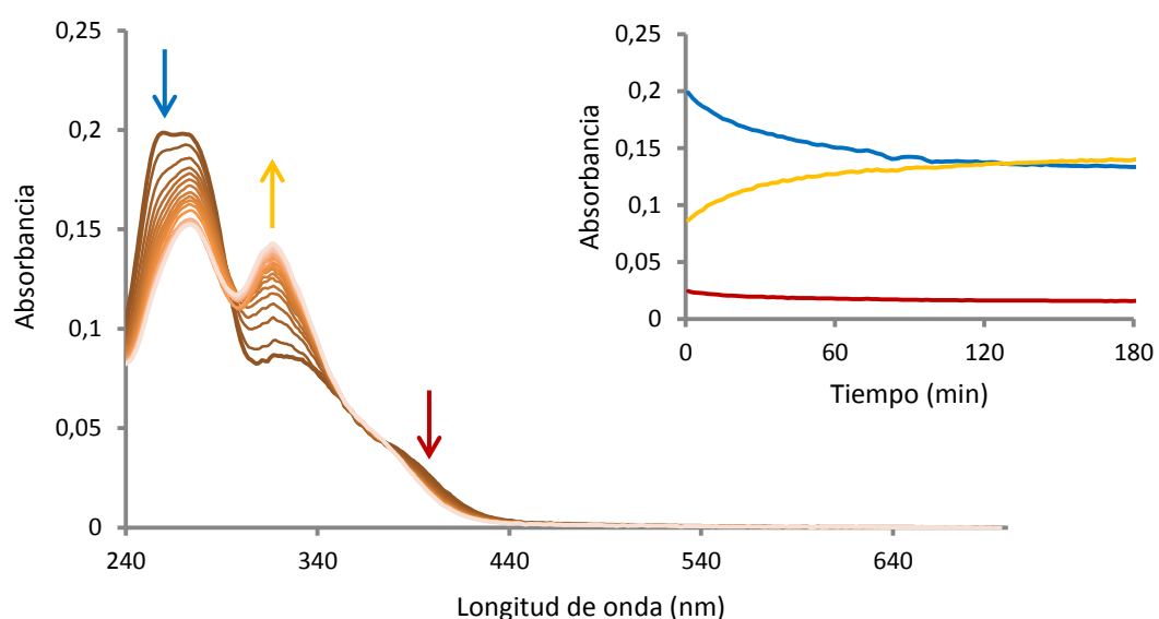
Figura 133 – Evolución temporal del espectro UV-Vis del compuesto 104 ( 5,0 \times 10^{-6} M, PBS/1% DMSO) al de ser tratado con un equivalente de TCEP ( 5,0 \times 10^{-6} M). El inserto de la esquina superior derecha muestra la evolución la absorbancia en función del tiempo transcurrido a 260 nm (azul), 320 nm (amarillo) y 400 nm (rojo).
