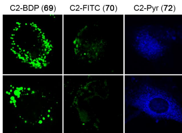
Figura 75 – Micrografías de microscopía confocal después del tratamiento de las líneas celulares U87MG (arriba) y NIH3T3 (abajo) con las tres sondas fluorescentes a una concentración 10 \mu\text{M} durante 1 hora a 37 ^{\circ}\text{C} .
