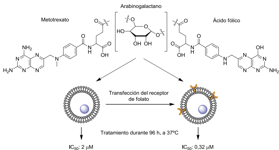
Figura 100 – Estructura del conjugado de metotrexato y ácido fólico donde se indican los valores de IC_{50} obtenidos en presencia o ausencia del receptor de folato. Se ha omitido en la representación la estructura del compuesto citotóxico y del sistema de liberación por claridad. 157
