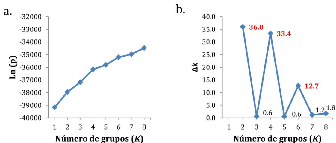
Figura 3.12 Gráficas del Ln de la probabilidad (a), y (b) \Delta K , del análisis de estructura poblacional de 38 poblaciones de maíz mexicanas. Se graficaron los valores promedio de \ln[\text{prob}(\text{dato})] de 5 corridas independientes para cada valor de K, de la misma manera estos valores fueron utilizados para el cálculo de los valores \Delta K . Con color rojo están marcados los más altos valores encontrados para \Delta K .
