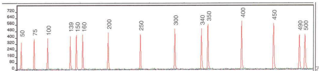
Figura 3.8 Patrón de fragmentos del estándar interno GS500 ROX bajo condiciones de desnaturalización.
