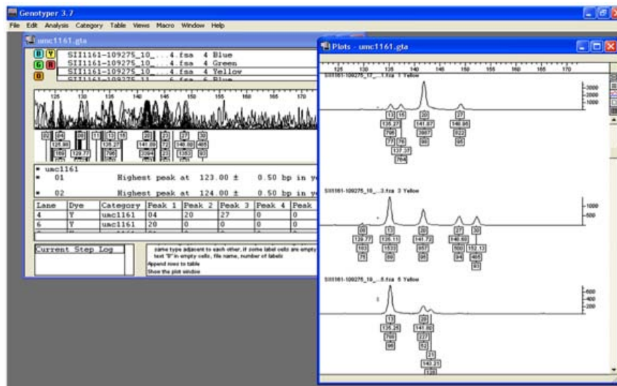
Figura 3.9 Identificación de fragmentos utilizando programa Genotyper® 2.1 (Applied Biosystems).
