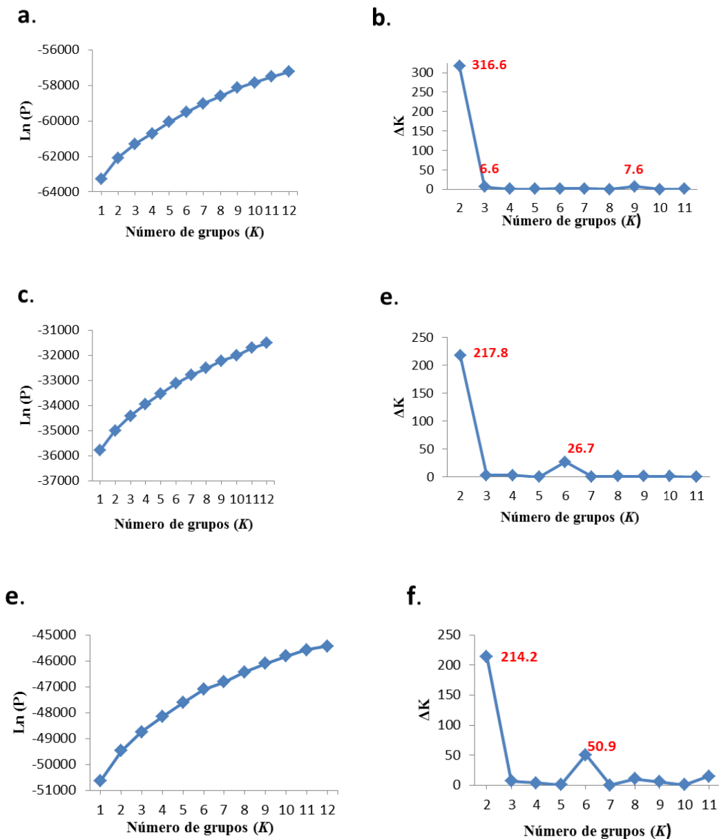
Figura 4.4 Gráficas del Logaritmo de la probabilidad y \Delta K para el análisis de estructura poblacional, (a) y (b) para panel inicial de 70 accesiones; (c) y (d) para panel seleccionado de 40 accesiones, (e) y (f) para solo poblaciones nativas, y (g) y (h) para nativas en el panel seleccionado. Se graficaron los valores promedios de \ln[\text{prob}(\text{dato})] de 3 corridas independientes para cada valor de K , de la misma manera estos valores fueron utilizados para el cálculo de los valores \Delta K . Con color rojo están marcados los valores más altos encontrados para \Delta K .
