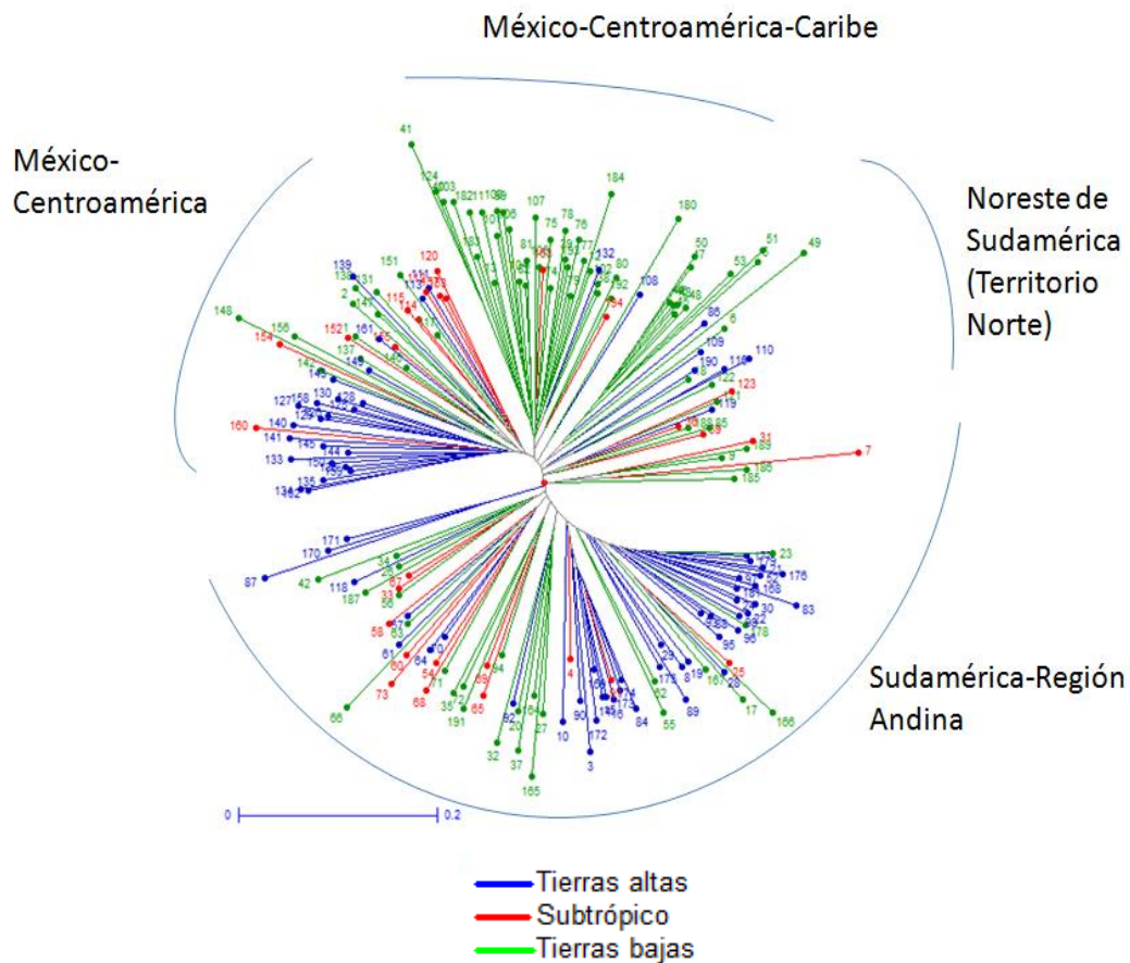
Figura 3.14 Análisis de agrupamiento para 194 poblaciones de maíz identificadas con número ID, provenientes de México, Centroamérica, Caribe y Sudamérica generado con el método Neighbor-Joining y basado en la distancia genética de proporción de alelos compartidos para 28 SSRs. Los colores denotan las distintas altitudes de las zonas de recolección de germoplasma.
