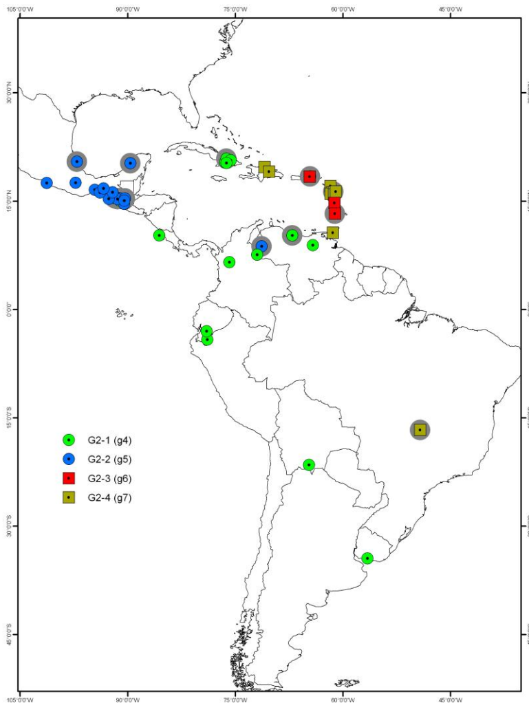
Figura 3.22 Distribución geográfica de las poblaciones del grupo G2 de acuerdo al análisis de subestructura poblacional ( Q > 51,0\% ), las poblaciones sombreadas con gris son las poblaciones menos representativas de los subgrupos ( 51,0\% < Q < 71,0\% )
