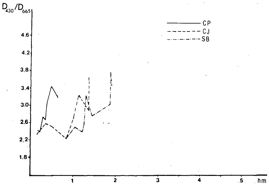
Fig. 10.- Valores del índice D_{430}/D_{665} con respecto a la altura sobre el nivel del mar en Can Picafort, Colònia de Sant Jordi y Son Bauló.
