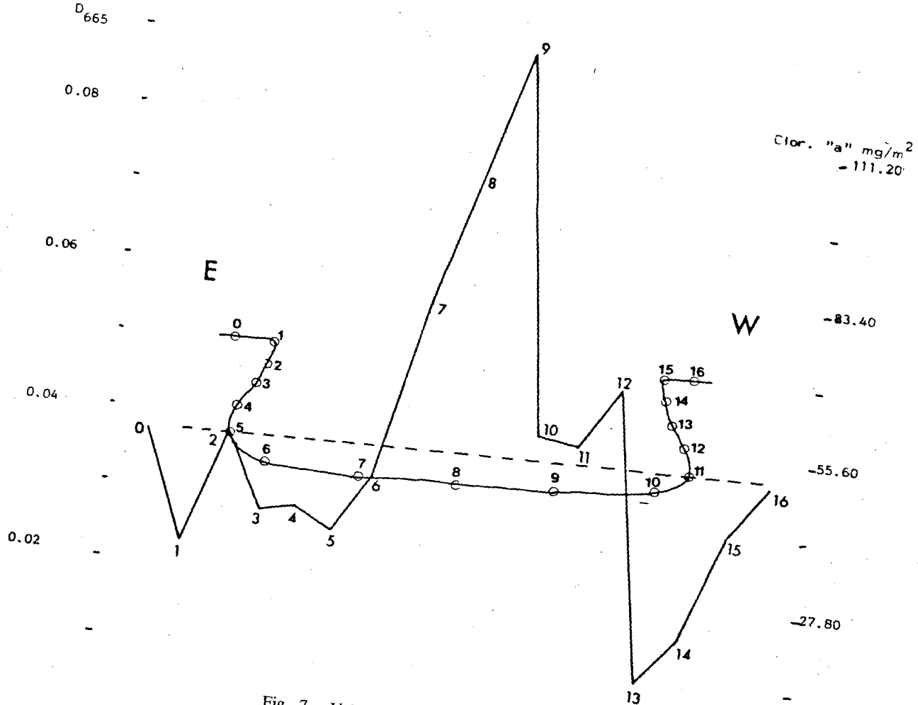
Fig. 7.- Valores de clorofila "a" en la cubeta.
