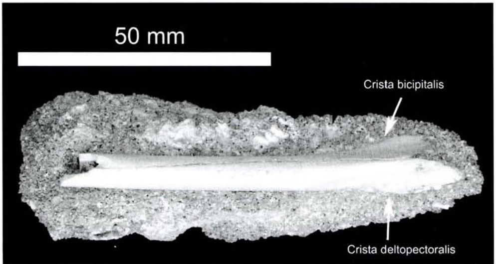
Fig. 3. Fragmento fósil de húmero en su aspecto caudal. Las flechas indican los márgenes de la Crista deltopectoralis y bicipitalis. Escala 50 mm.
