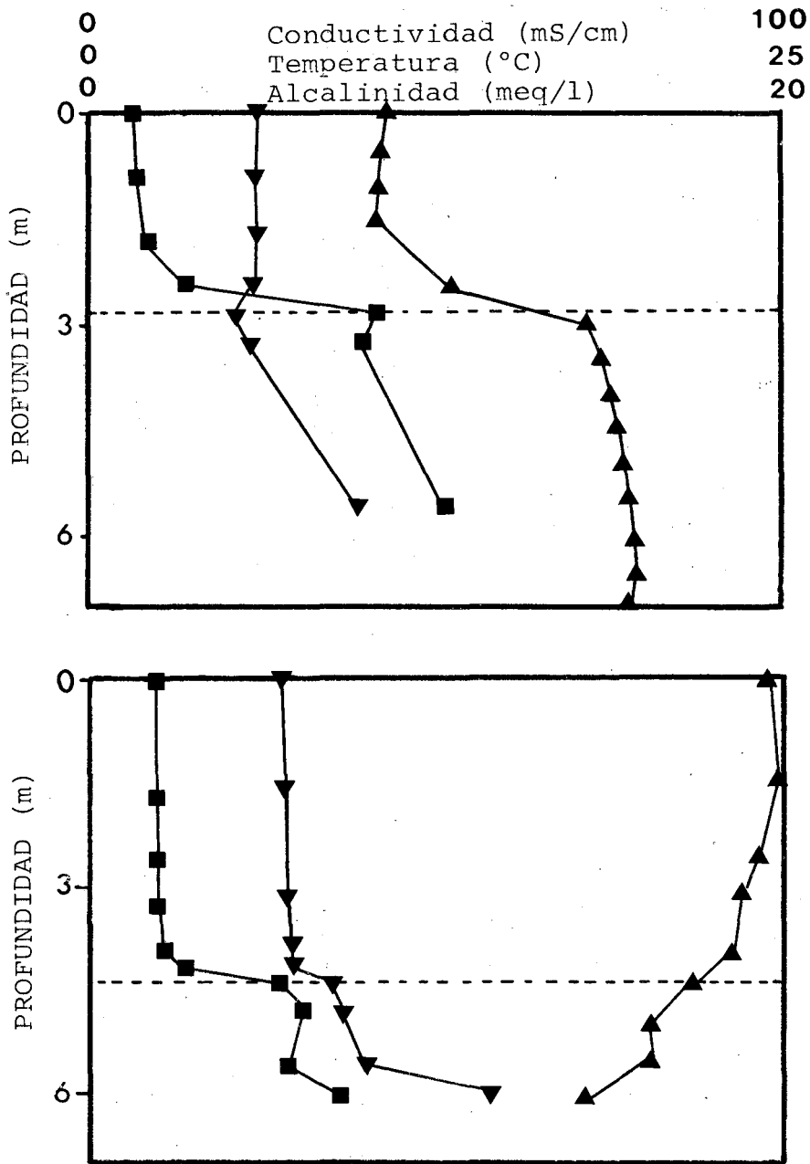
Fig. 1.- Distribución vertical de la alcalinidad (▼), temperatura (▲) y conductividad (■), y situación de la quimioclina en dos periodos estacionales distintos, octubre de 1986 (gráfica superior) y junio de 1987 (gráfica inferior).
