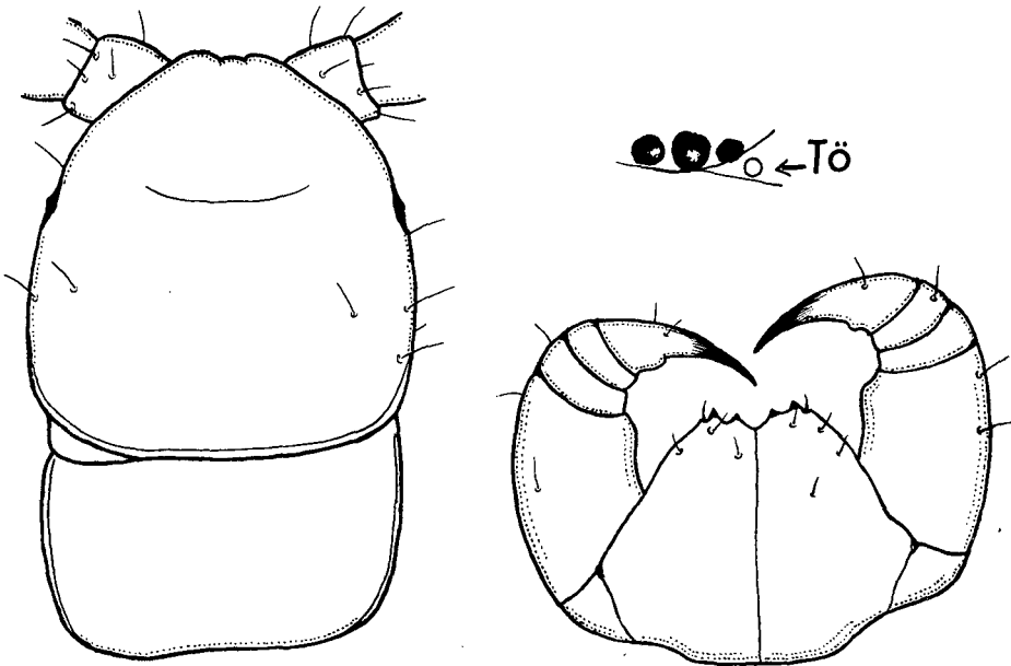
Fig. 5.— Lithobius (M.) georgescui n. sp. La tête vue du côté dorsal, les ocelles et les forcipules.
