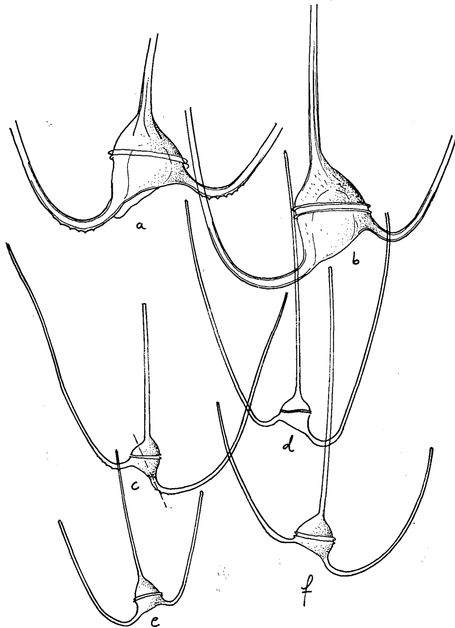
Fig. 6-a: Ceratium massiliense .
