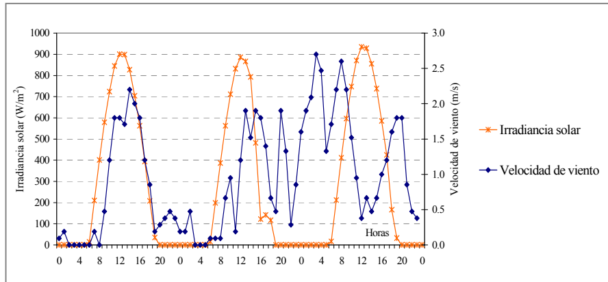
Figura 8: Irradiancia solar sobre superficie horizontal y velocidad del viento
