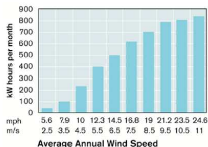
Figura 8: Curva de potencia aerogenerador de 1,9 Kw. Modelo: Skystream 3.7: Fabricante: Southwest Windpower
