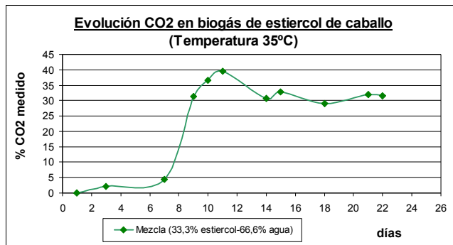
Figura 4: Niveles de dióxido de carbono medidos en el biogás producido
