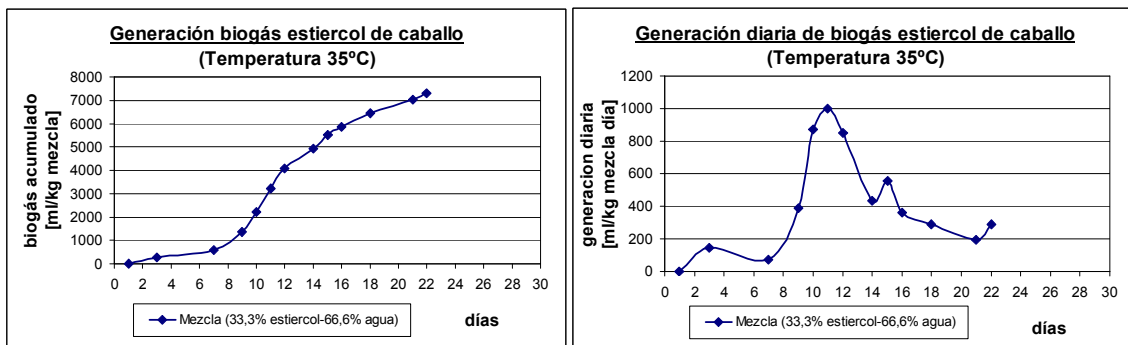
Figura 3: Generación acumulada de biogás del estiércol de equino y producción diaria a 35°C.
