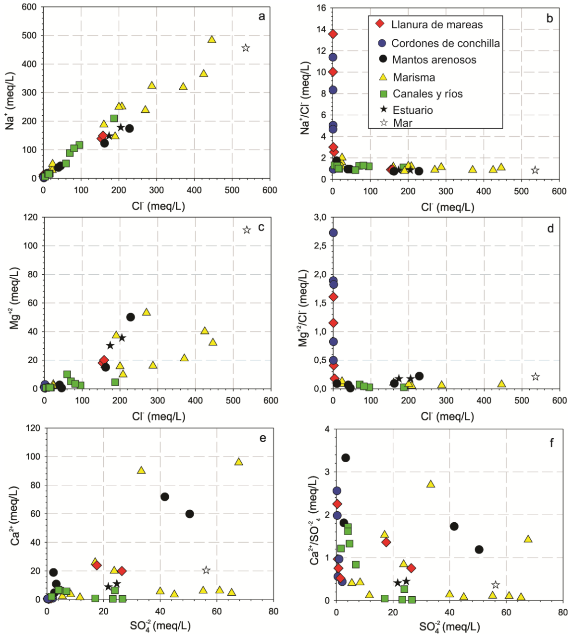
Figura 2. Relaciones iónicas.
