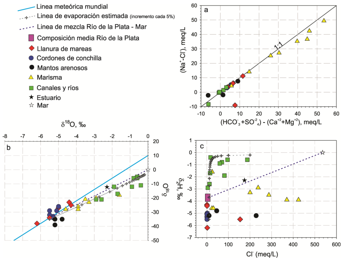
Figura 3. Relaciones iónicas e isotópicas.
