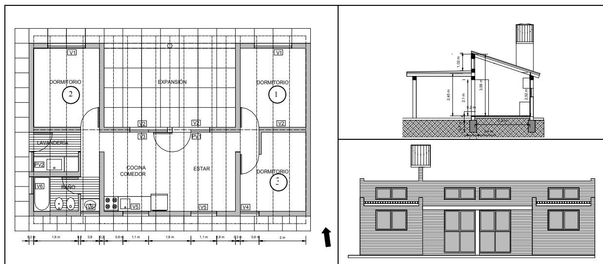
Figura 1: Planta, corte y vista Norte de la vivienda
