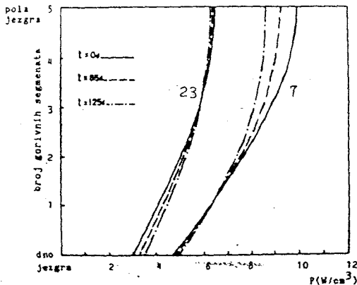
Slika 3. Aksijalna raspodela gustine snage u donjoj polovini jezgra reaktora RA u zavisnosti od izgaranja (7 i 23 odgovaraju položajima gorivnih elemenata u pravcu R kao na slici 2.)
