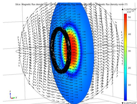
Gambar 3. Bentuk Kerapatan Fluks Medan Magnetik (B) dengan potongan vertikal
