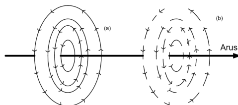
Gambar 1. Dua cara untuk menggambarkan medan magnetik dari sebuah kawat lurus yang membawa arus: (a) garis-garis medan, dimana kedekatan setiap garis menunjukkan intensitas medan; dan (b) gambar vektor, dimana arah dan besaran setiap vektor menunjukkan arah dan intensitas medan pada setiap titik. Setiap titik garis medan mempunyai arah yang sama seperti vektor medan [8].
