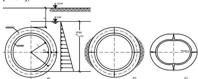
Bild 3: Lastfälle des Inliners; Grafik aus [Fal94] a) undichtet Altrhr, allein tragfähig (Zustand I), b) Altrhr-Boden-System tragfähig (Zustand II), c) Altrhr-Boden-System nicht allein tragfähig (Zustand III)
