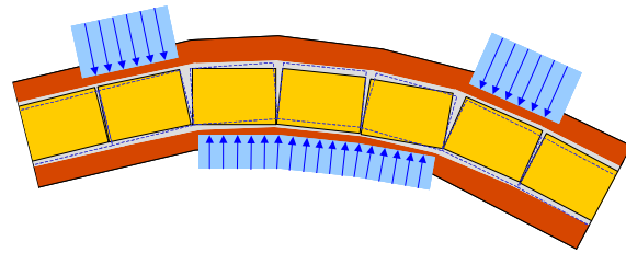
Bild 2: Versuchsergebnisse: Qualitative Kontaktspannungsverteilung; aus [IKT07]
