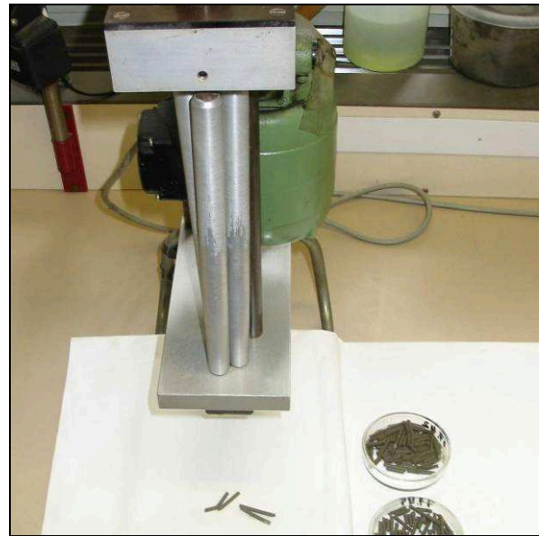
Bild 8: Gerät zur Bestimmung der Ausrollgrenze
