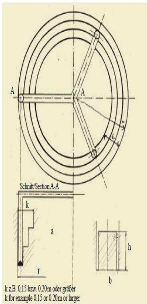
Bild 1: Abmessung Bohrlochrand-Schmelze
