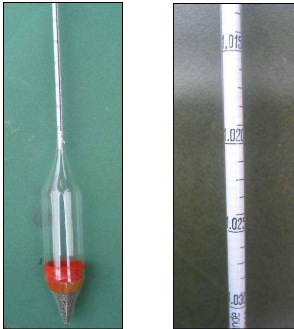
Bild 3: Aräometer mit Detail Ablesekala
