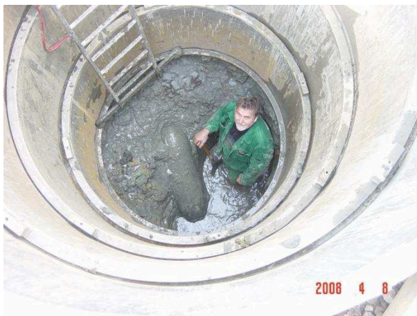
Bild 8: Bombenfund in einem Ringverbau Quelle Fa. Schollenberger 2008
