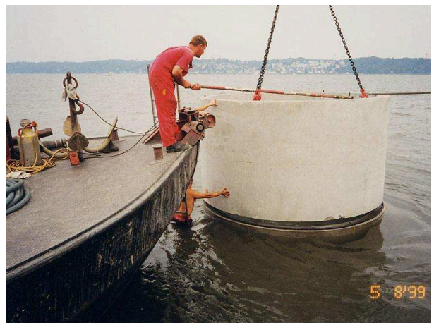
Bild 13: Einsatz eines Spezialverbaues für die Gewässersondierung Quelle Fa, Hirdes 1999
