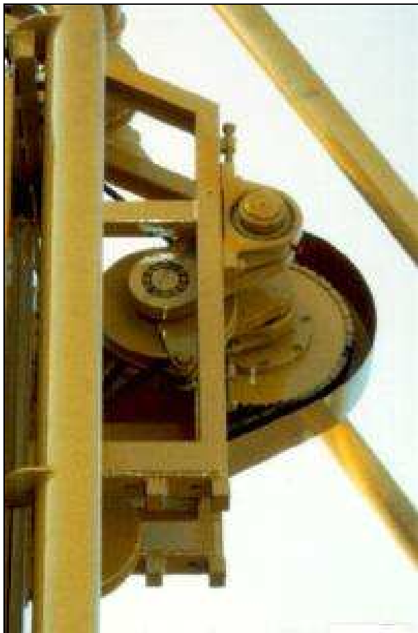
Bild 10: Freifall-Seilschlagvorrichtung
