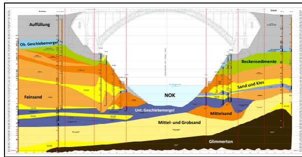
Bild 7: Profilschnitt Levensauer Hochbrücke
