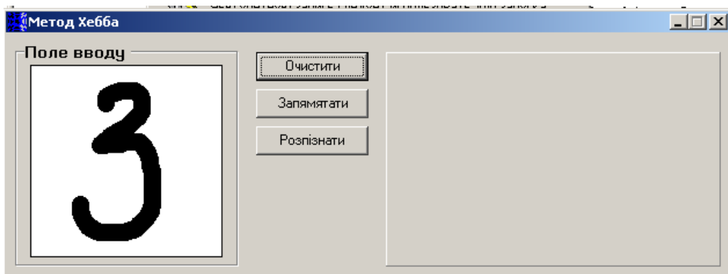
Рисунок 3.13 - Ввід цифри «3»
