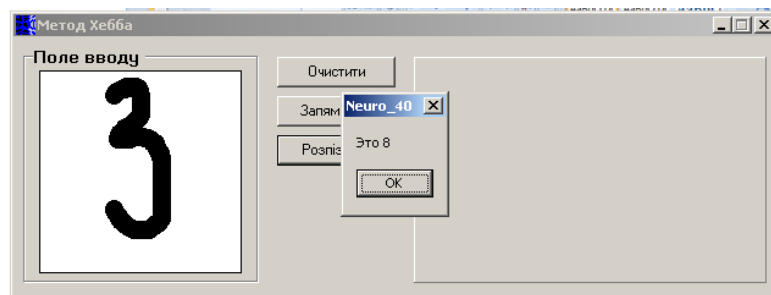
Рисунок 3.11 - Розпізнавання цифри «3»
