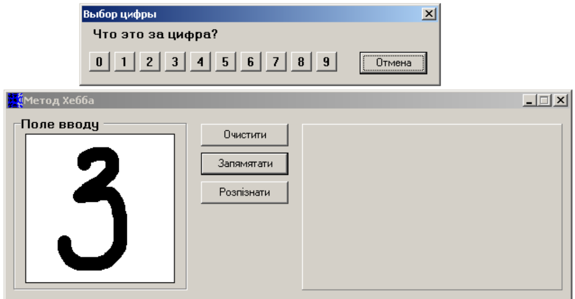
Рисунок 3.8 - Навчання цифри «3»
