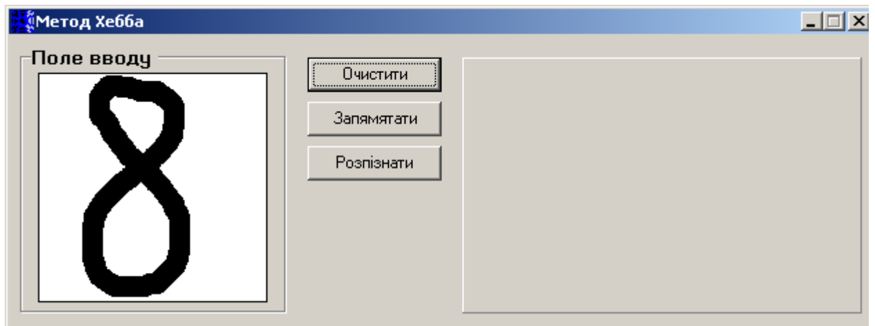
Рисунок 3.9 - Ввід цифри «8»
