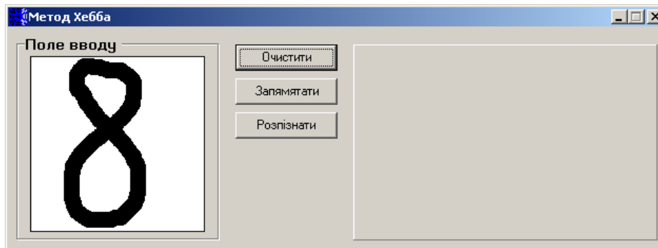
Рис. 3.12. Ввід цифри «8»
