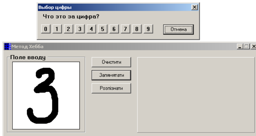
Рисунок 3.14 - Навчання цифри «3»
