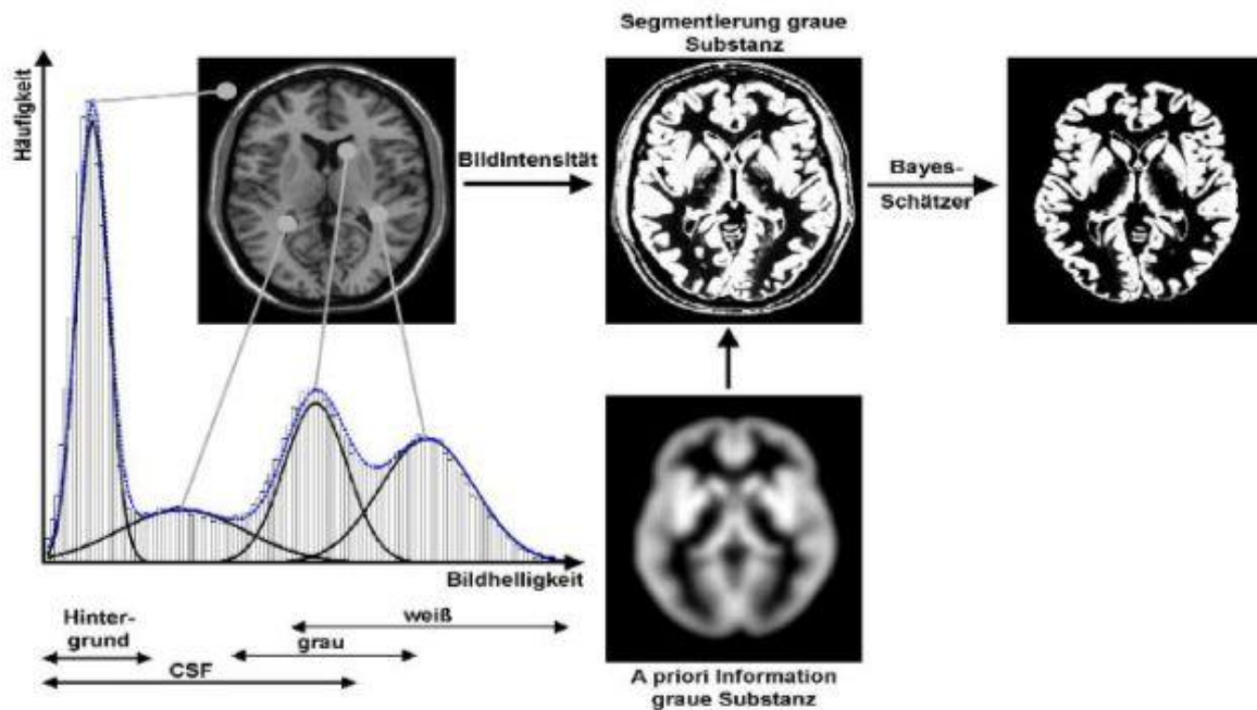
Abb. 4 Segmentierung. Die Segmentierung eines Bildes in graue und weiße Substanz und CSF ist hier dargestellt am Beispiel eines Gaussian-Mixture-Model in Verbindung mit einem Expectation-Maximization-Algorithmus. Dabei wird nicht nur die Information der Bildintensität genutzt, sondern zusätzlich geht auch die A-priori-Information über die räumliche Verteilung für graue und weiße Substanz und CSF ein. Die Häufigkeit der einzelnen Bildintensitäten über das gesamte Bild bildet das Histogramm, in das einzelne Gaußkurven für die jeweiligen Verteilungen eingepasst werden. Zusätzlich zu dieser Helligkeitsinformation wird eine A-priori-Information aus bereits segmentierten Gehirnen verwendet und über einen Bayes-Schätzer verknüpft. CSF=Liquor. Bild aus (Gaser, 2005)
