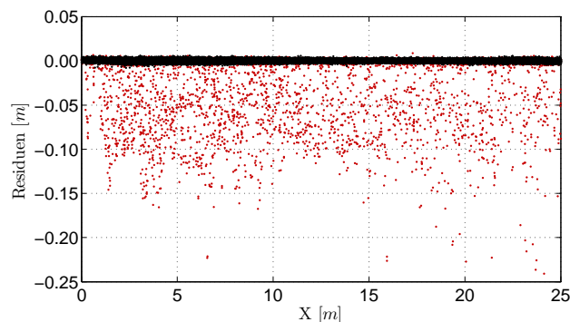
Abbildung 5.12: Klassifizierung der Residuen vom Ausgleich nach ihrer Position (schwarz = innerhalb Paneel, rot = zwischen Paneelen).
