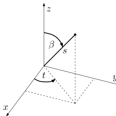
Abbildung 3.7: Polarbeobachtungen s, \beta, t und kartesische Koordinaten x, y, z im Scannersystem.
