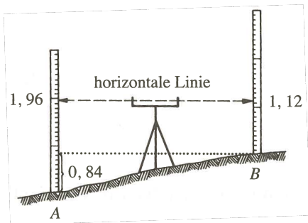
Abbildung 3.1: Methodik des Nivellements zur Bestimmung des Höhenunterschieds h_{AB} = 1.96 \text{ m} - 1.12 \text{ m} = 0.84 \text{ m} zwischen zwei Punkten A und B [Kahmen, 2006, S. 401].
