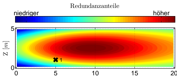
Abbildung 5.7: Redundanzanteile beim Scanning einer Ebene von Standpunkt 1 nach Punktausdünnung.
