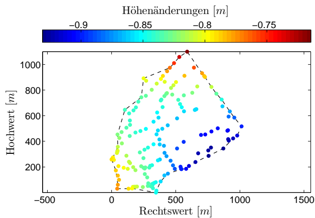
Abbildung 3.3: Punktverteilung und Höhenänderungen (farblich codiert) beim Nivellement in der Beispielregion B.
