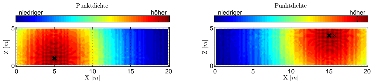
Abbildung 3.8: Relative Punktdichte nach Abtastung mit Hilfe eines terrestrischen Laserscanners von den Standpunkten 1 und 3 in 10 m Entfernung zur Ebene; Simulation auf Basis einer gescannten Ebene (schwarzes Kreuz = Projektion des Scannerstandpunktes in Ebene).
