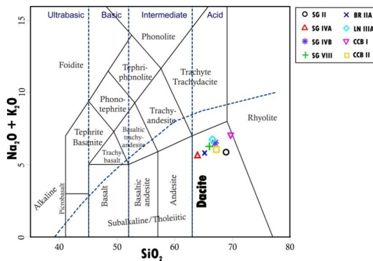
Gambar 6. Plotting \text{Na}_2\text{O} + \text{K}_2\text{O} vs \text{SiO}_2 dalam diagram TAS Le Bas et al., 1986 menunjukkan batuan yang diteliti jenis dasit dari Kompleks Mélange Luk Ulo.
