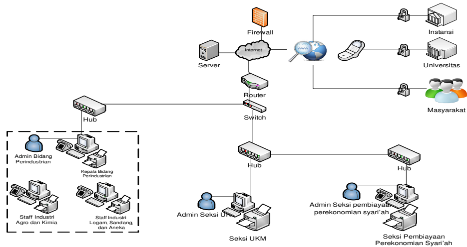
Gambar 4.21 Arsitektur Infrastruktur Jaringan
