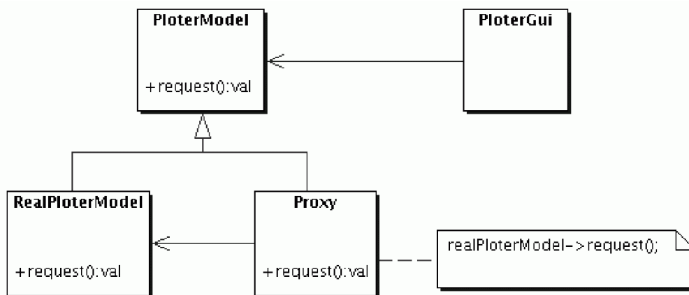
Fig. 4.8 - Padrão Proxy implementando o controle de concorrência.
