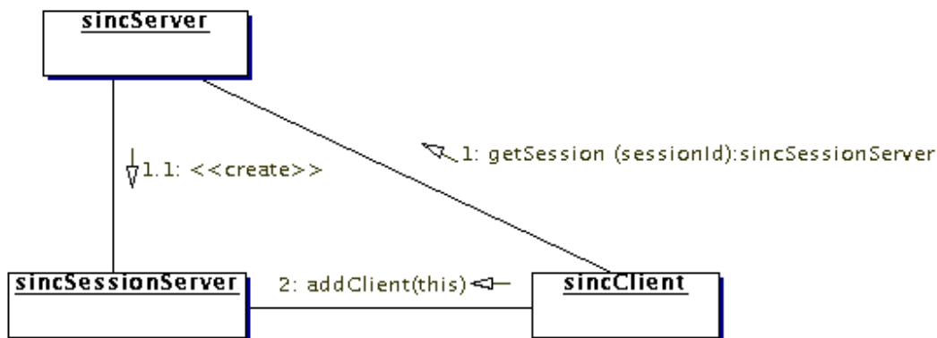
Fig. 3.7 - Diagrama de colaboração mostrando a conexão do cliente com o servidor da ferramenta de comunicação genérica.
