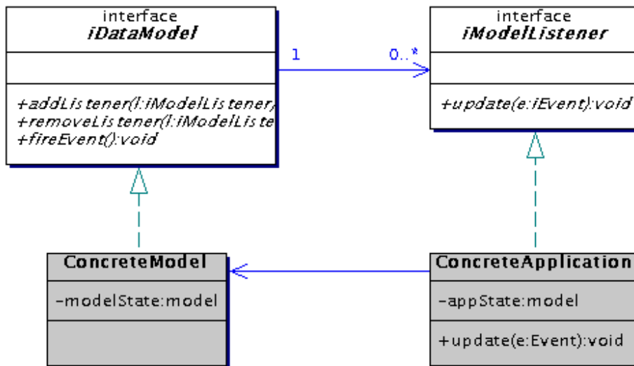
Fig. 3.5 - Classes concretas implementando o modelo de dados e aplicação de visualização.
