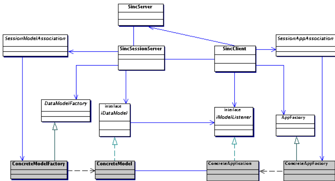
Fig. 3.10 - Modelo completo da arquitetura proposta.
