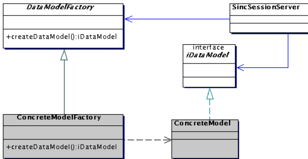
Fig. 3.9 - Classes concretas implementando o modelo de dados e aplicação de visualização.
