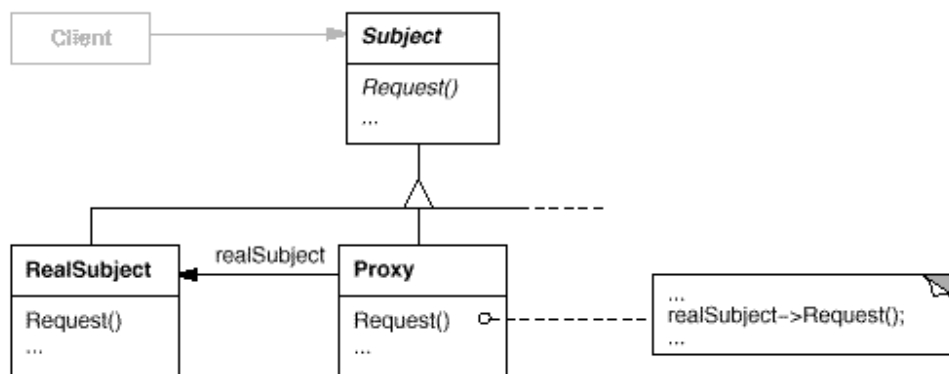
Fig. 2.3 - Padrão proxy
