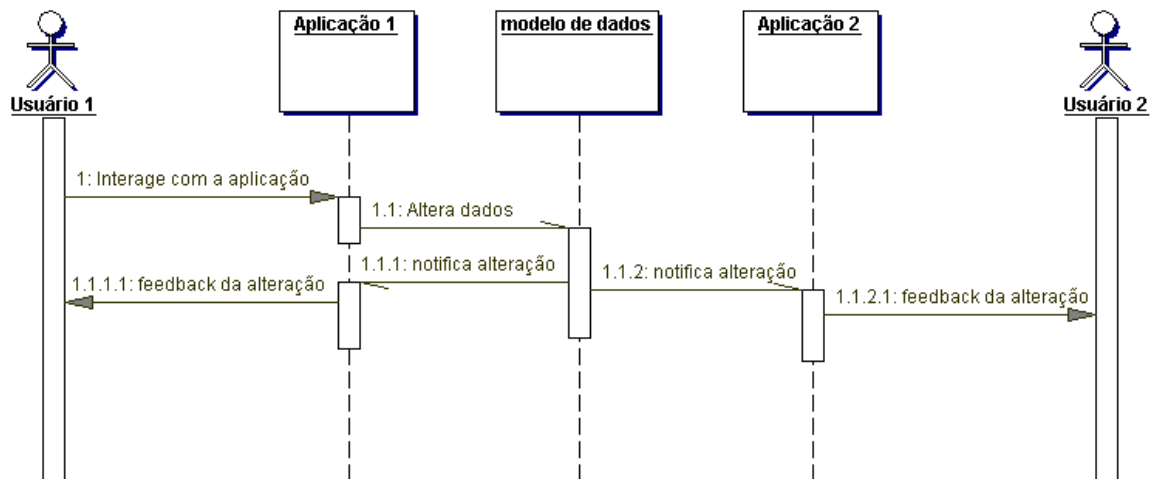
Fig. 3.3 - Broadcasting da alteração no modelo de dados.
