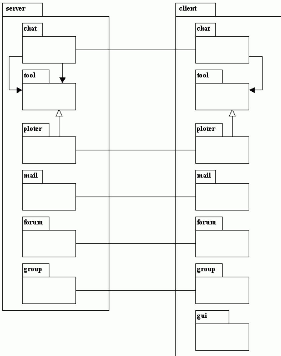
Fig. 4.1 - Divisão das classes do CoLab em pacotes
