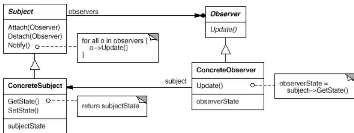
Fig. 2.1 - Padrão observer .
