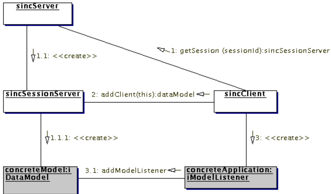
Fig. 3.8 - Diagrama de colaboração mostrando como a ferramenta de comunicação inicializa a aplicação gráfica.
