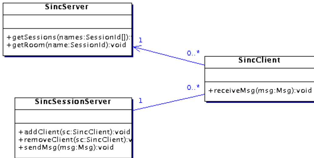
Fig. 3.6 - Classes implementando um modelo cliente-servidor para uma ferramenta de comunicação genérica.
