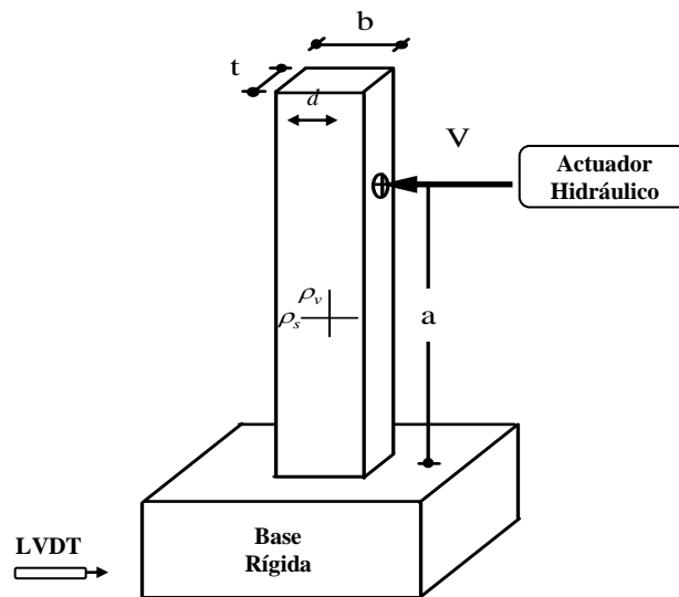
Figura 5. Esquema de aplicación de desplazamientos impuestos en las probetas de ensayo. Fuente: los autores
