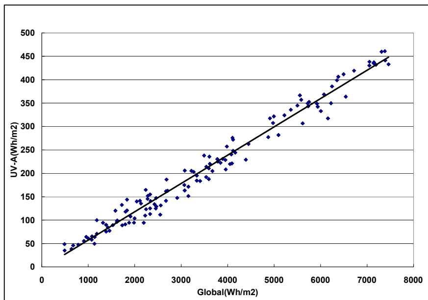
Figura 1. Correlación entre irradiación Global y UV-A para la ciudad de Buenos Aires.
