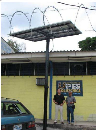
Figura 6. Generador fotovoltaico del SFCR
