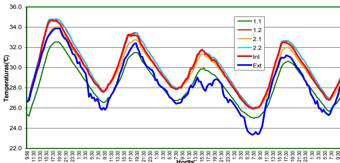
Fig.4 – Temperaturas internas y externa según los distintos sensores entre las 10:00hs del 05/01/2004 y las 11:00hs del 09/01/2004
