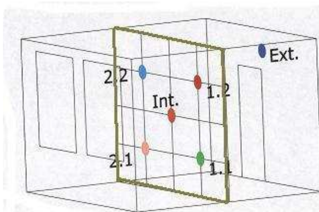
Fig. 3 - Ubicación de los sensores en el plano medio del recinto
