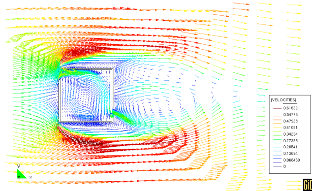
Fig. 8. Campo de vectores de velocidad (instantes finales).
