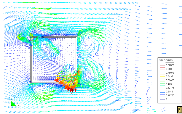
Fig. 7. Campo de vectores de velocidad (instantes iniciales).
