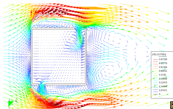
Fig. 15. Distribución de velocidades (instantes finales).
