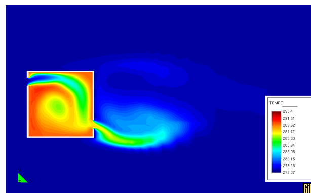
Fig. 10. Distribución de temperatura (instantes finales).
