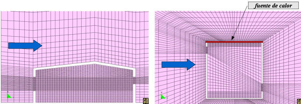
Fig. 1. Mallado, vista de perfil, 6386 nodos - 6148 elementos
