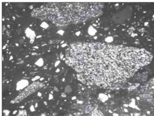
Figura 5. Fotomicrografía en nicoles cruzados (80x) de un sector de la pasta del fragmento Ordinario Tumi B1 15.2-8 (muestra 2) mostrando las metamorfitas típicas de la Formación Puncoviscana.
