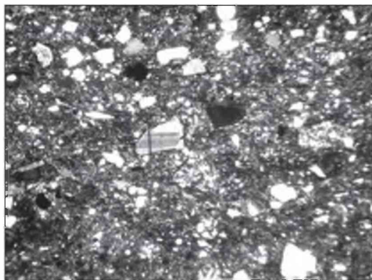
Figura 3. Fotomicrografía en nicoles paralelos (80x) de la pasta característica de los Pucos Bruñidos. Inclusiones no plásticas de andesita, cuarzo, plagioclasa y hornblenda.
