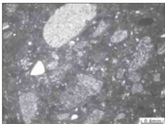
Figura 7. Fotomicrografía en nicoles cruzados (80x) de un sector de la pasta del plato Yavi/Chicha Ante liso (muestra 4).
