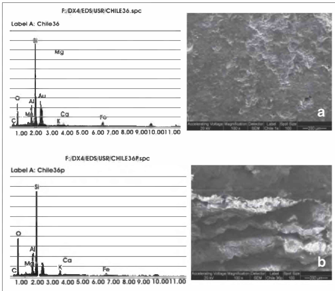
Figura 10. SEM-EDAX. a) Composición y fotomicrografía (520x) de la superficie de un puco rojo pulido del Grupo 36 de Turi; y b) Composición y fotomicrografía (520x) de la pasta del mismo puco.
