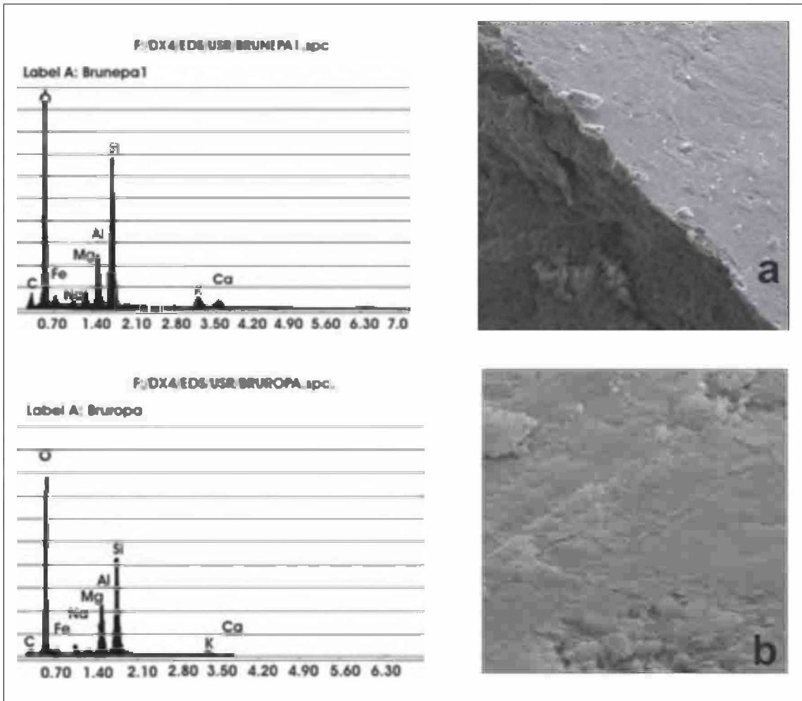
Figura 9. SEM-EDAX. a) Composición y fotomicrografía (520x) de la pasta del Puco Bruñido rojo Tumi B1 24.11-5, y b) Composición y fotomicrografía (520x) de la superficie externa del mismo puco en la que se observan las líneas de pulimento.
