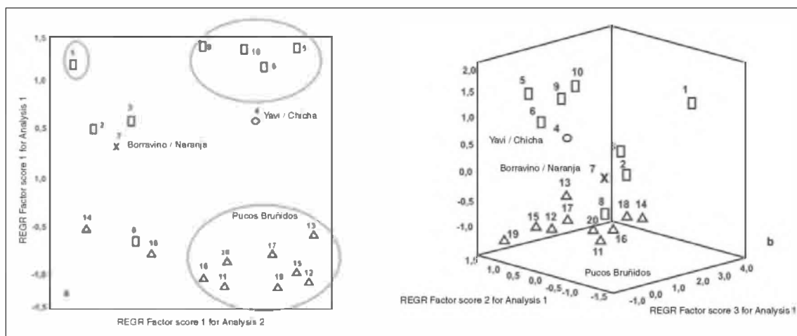
Figura 11. Análisis de componentes principales (Programa SPSS 11.0.1). a) Proyección en 2D; b) Proyección en 3D de los primeros componentes calculados a partir de las concentraciones de los elementos traza determinadas por ICP-MS. Referencias: \Delta : Pucos Bruñidos, \square 1 y 2: Ordinario, 3: Aríbalo Castaño, 6: Negro Pulido, 5 y 8: Humahuaca N/R, 9 y 10: Humahuaca Inca. \circ : Yavi/Chicha, X: Borravino/Naranja.
