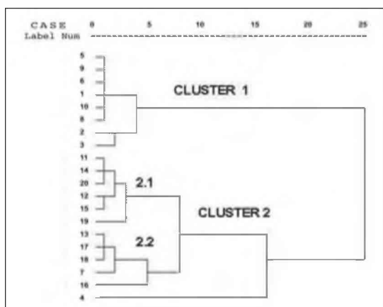
Figura 4. Análisis de agrupamiento ( cluster analysis ). Representación en un fenograma de las 20 secciones delgadas analizadas. Programa SPSS 11.01.
