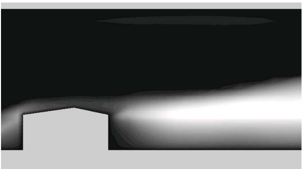
Figura 4: Energía cinética turbulenta modelo k - \epsilon ( Re = 8.1 \times 10^4 )
