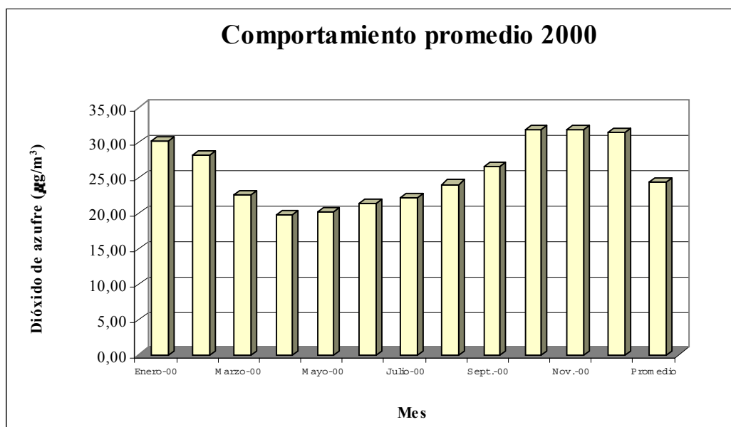
Figura 5. Concentración mensual promedio de dióxido de azufre en la zona industrial de la Ciudad de Santa Clara en el año 2000.
