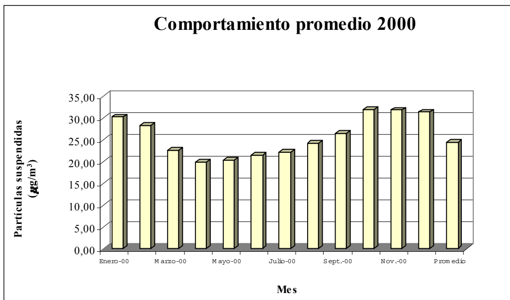
Figura 4. Concentración mensual promedio de partículas sólidas suspendidas en la zona industrial de la Ciudad de Santa Clara en el año 2000.
