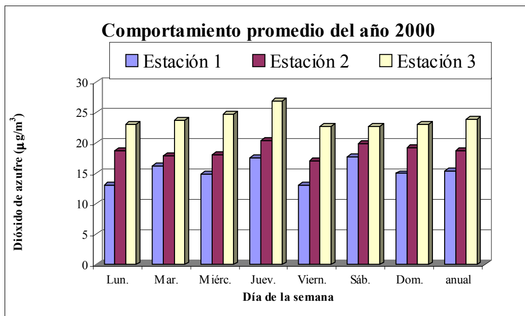
Figura 3. Concentración diaria promedio de dióxido de azufre en diferentes puntos de la Ciudad de Santa Clara en el año 2000.
