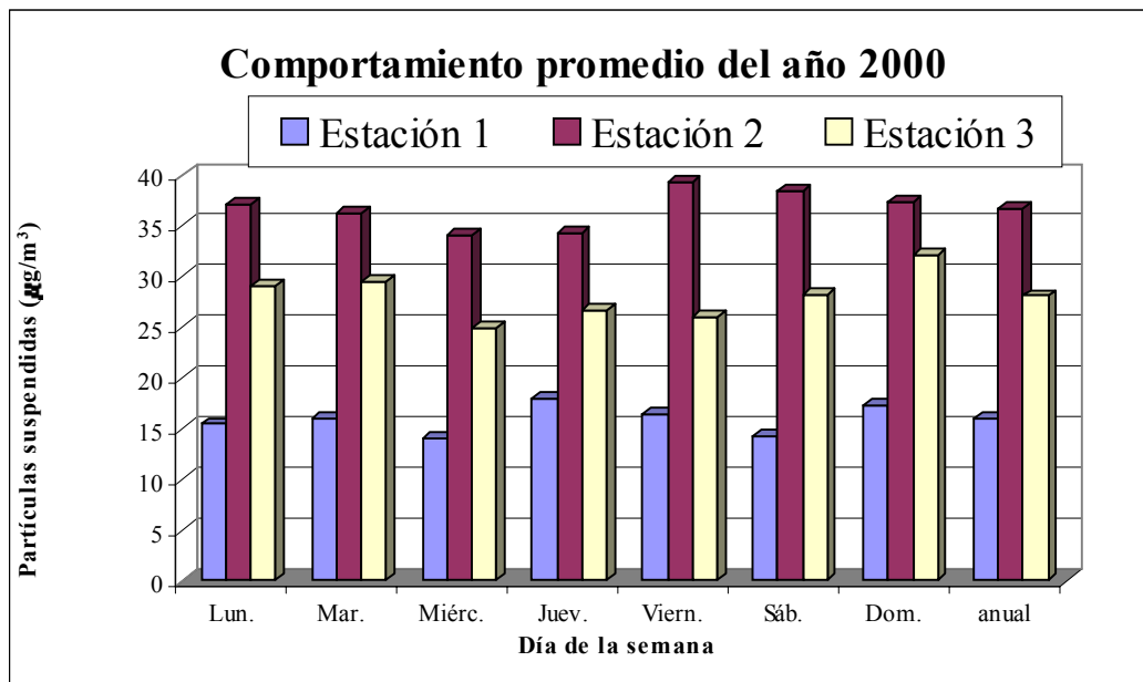
Figura 2. Concentración diaria promedio de partículas sólidas suspendidas en diferentes puntos de la Ciudad de Santa Clara en el año 2000.
