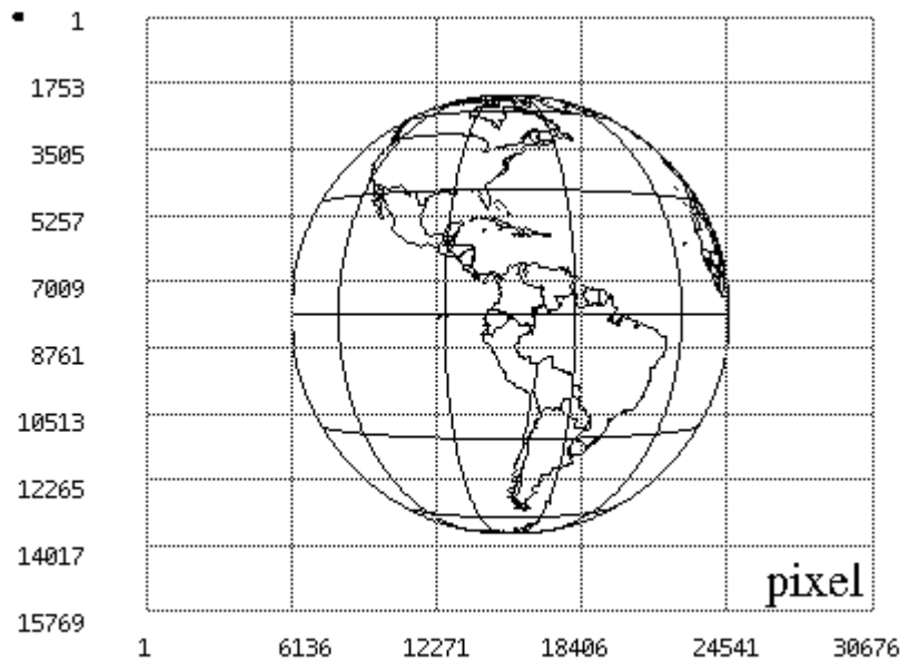
Figura 2: Sistema de coordenadas línea-píxel de GOES a 75 W.
