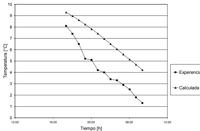
Figura 4: Temperaturas en el interior del invernadero
