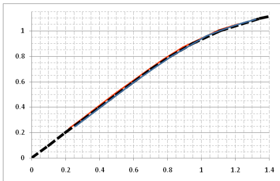
Fig. 1. Curva saturación Máquina Síncrona. Ensayos curvas azul/rojo, aprox. curva negra.
