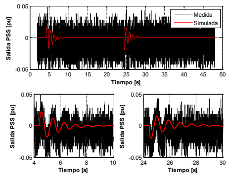
Fig. 14. Pulso +3 %, 20 s. Salida PSS. Sin PSS.
