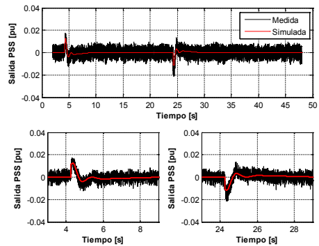
Fig. 12. Pulso +3 %, 20 s. Salida PSS. Con PSS.
