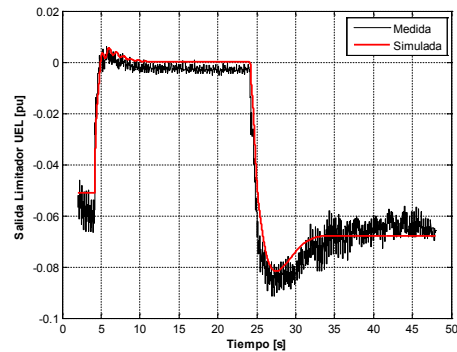
Fig. 8. UEL. Pulso -3 %, 20 s. Salida del Limitador.
