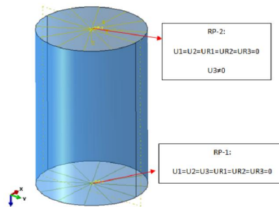
Figura 8. Condiciones de borde sobre el modelo FEM
