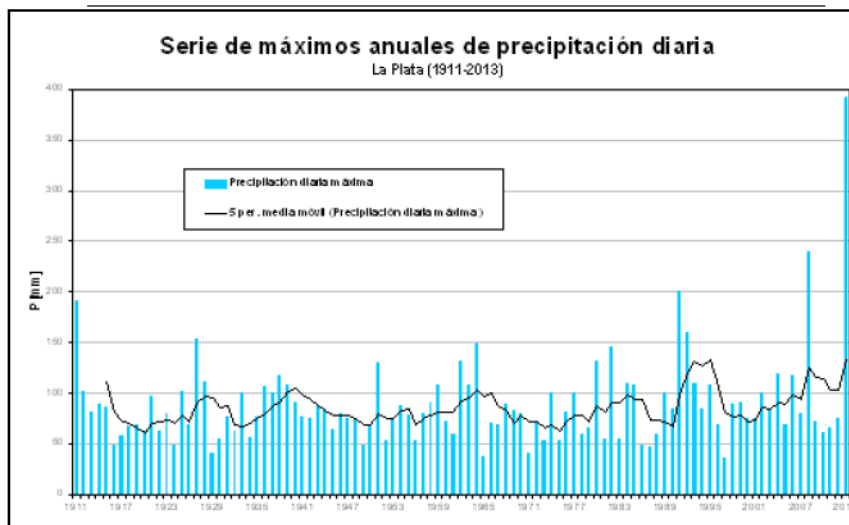
Figura 1–Serie de precipitaciones diarias máximas [mm] en el período 1911-2013
