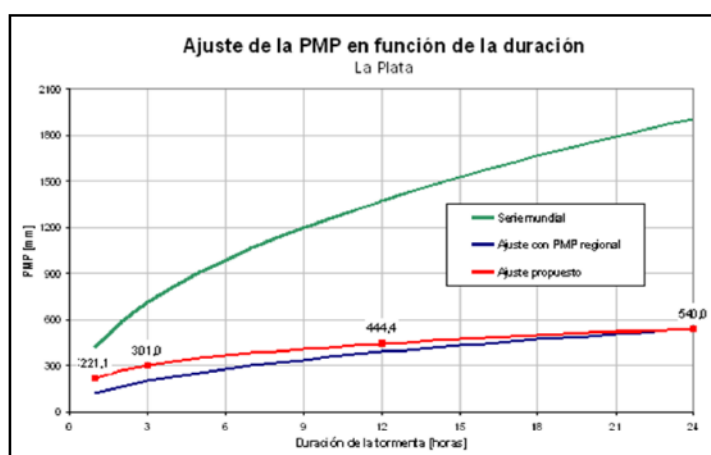
Figura 2 – Ajuste de la PMP [mm] para duraciones inferiores al día.
