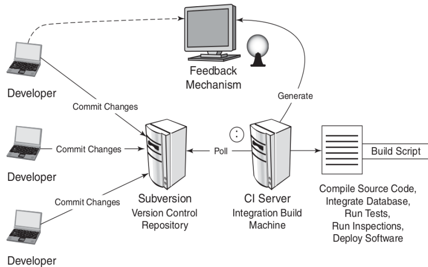
Fig. 1. Escenario típico de Integración Continua.
