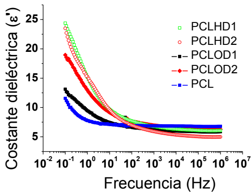
Figura 3. Constante dieléctrica.
