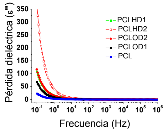
Figura 4. Pérdida dieléctrica
