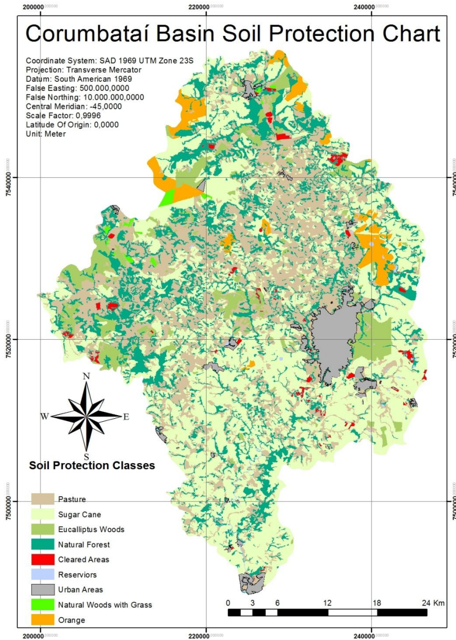
Figura 4. Unidades de graus de proteção do solo na Bacia do Corumbataí.
