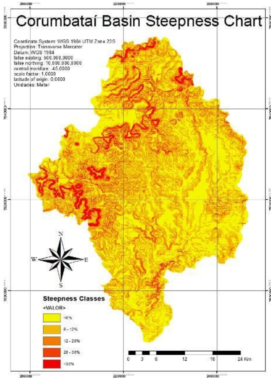
Figura 2. Carta de declividades para a Bacia do Corumbataí.
