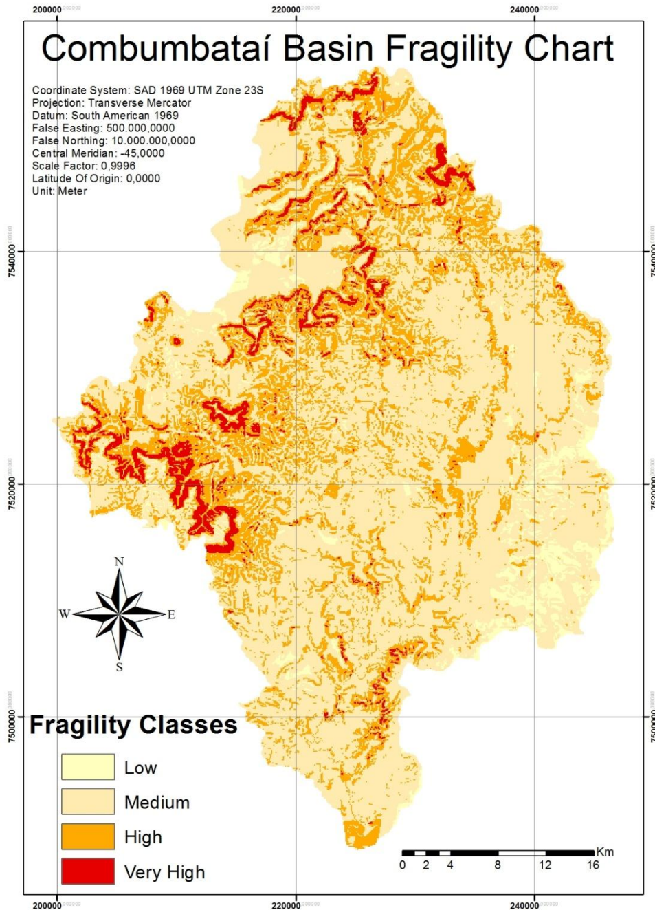
Figura 5. Carta de fragilidade ambiental para a Bacia do Corumbataí.
