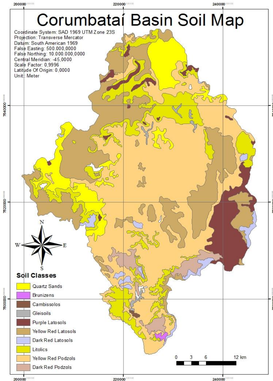
Figura 3. Mapa pedológico para a Bacia do Corumbataí.
