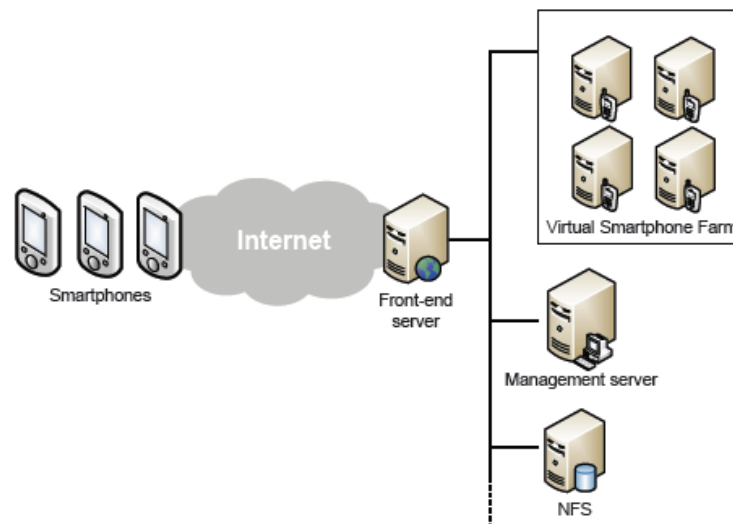
Figura 4 – Arquitectura de Smartphone virtual
